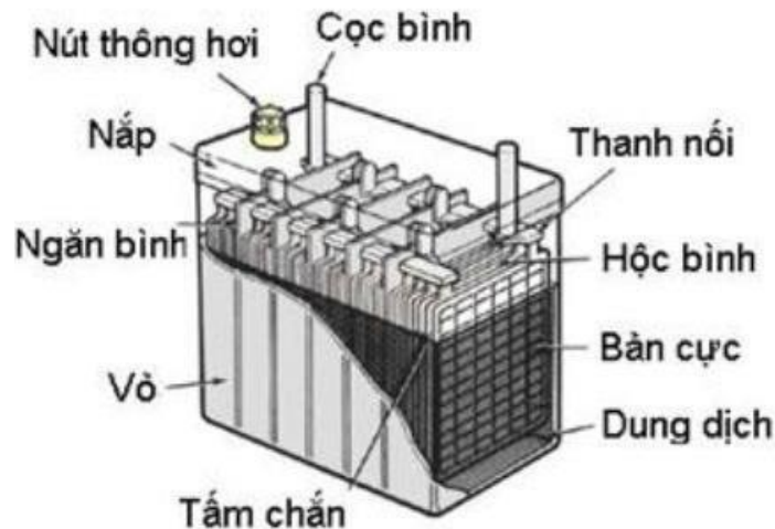
Hình 2.14 Cấu tạo của ắc quy
