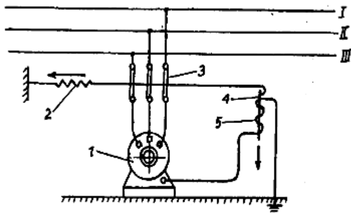
Hình 2-14 Cắt điện bảo vệ tự động
