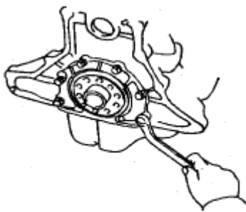
Tháo phôt chắn dầu
