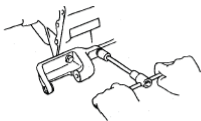
Lắp giá đỡ máy phát điện
