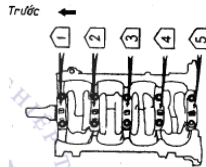
Lắp nắp gói đỡ trục khuỷu
