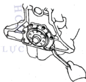
Bắt chặt giá đỡ phốt dầu
