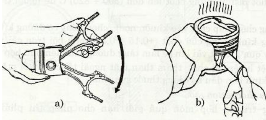
Hình 5.4. Kiểm tra độ kín khí của lỗ và chốt piston.
