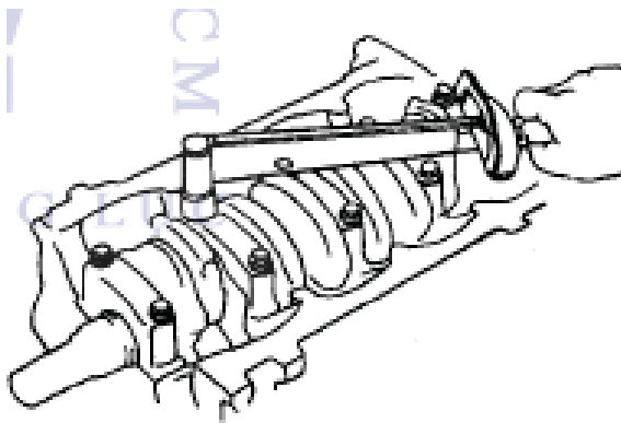
Siết bu lông gối đỡ
