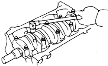
Tháo bu lông bắt gôỉ đỡ trục
