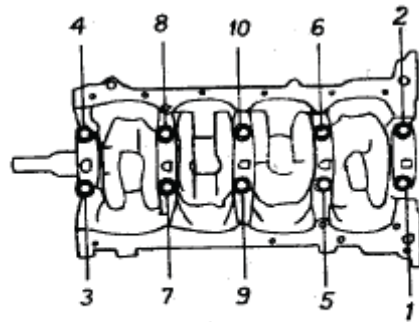
Trình tự nới bu lông
