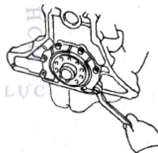
Bắt chặt giá đỡ phốt dầu
