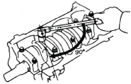
Siết bu lông thêm 90°
