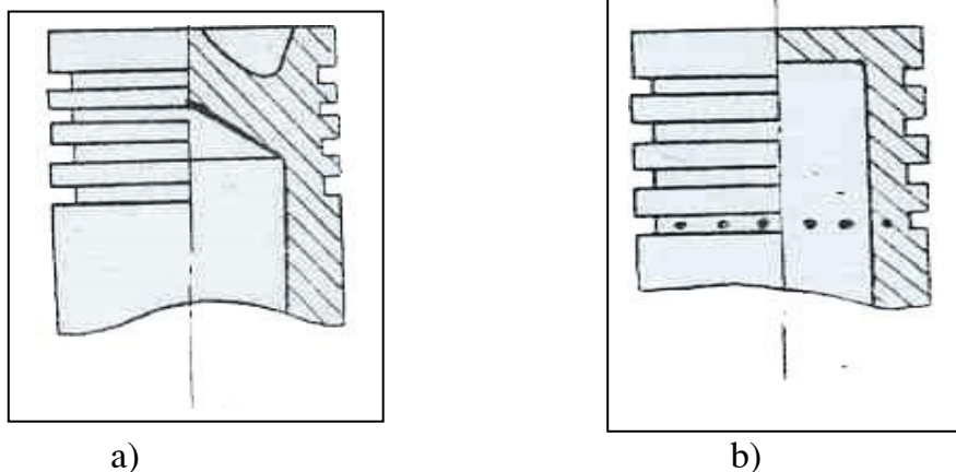
Hình 1.8. Các dạng đỉnh pít tông.
