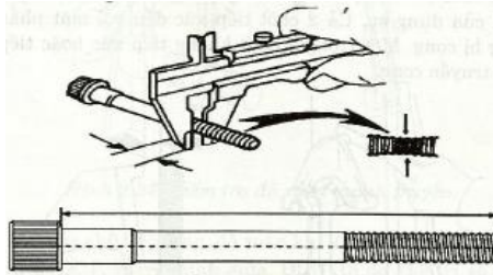
Hình 6.1. Kiểm tra bu lông thanh truyền
