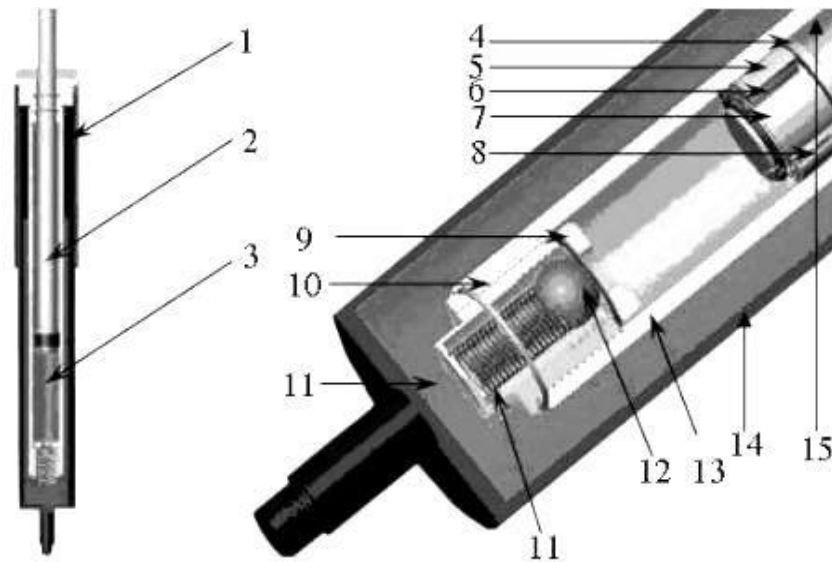
Hình 1.15. Cấu tạo chung của một ống giảm xóc
