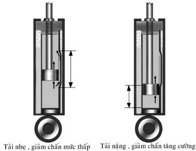
Hình 1.18. Giảm xóc Vario
