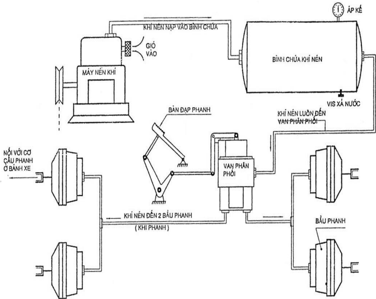
Hình 1.21 Sơ đồ hệ thống phanh khí ( không có Rơ-móc )
