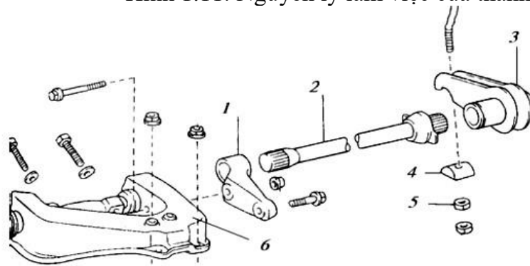
Hình 1.12. Kết cấu chung của bộ phận đàn hồi sử dụng thanh xoắn 1. Giá xoay; 2. Thanh xoắn; 3. Giá cố định; 4. Đệm điều chỉnh; 5. Đai ốc điều chỉnh; 6. Đòn treo trên.
