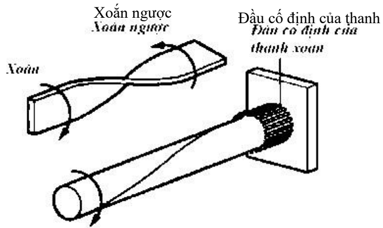
Hình 1.11. Nguyên lý làm việc của thanh xoắn
