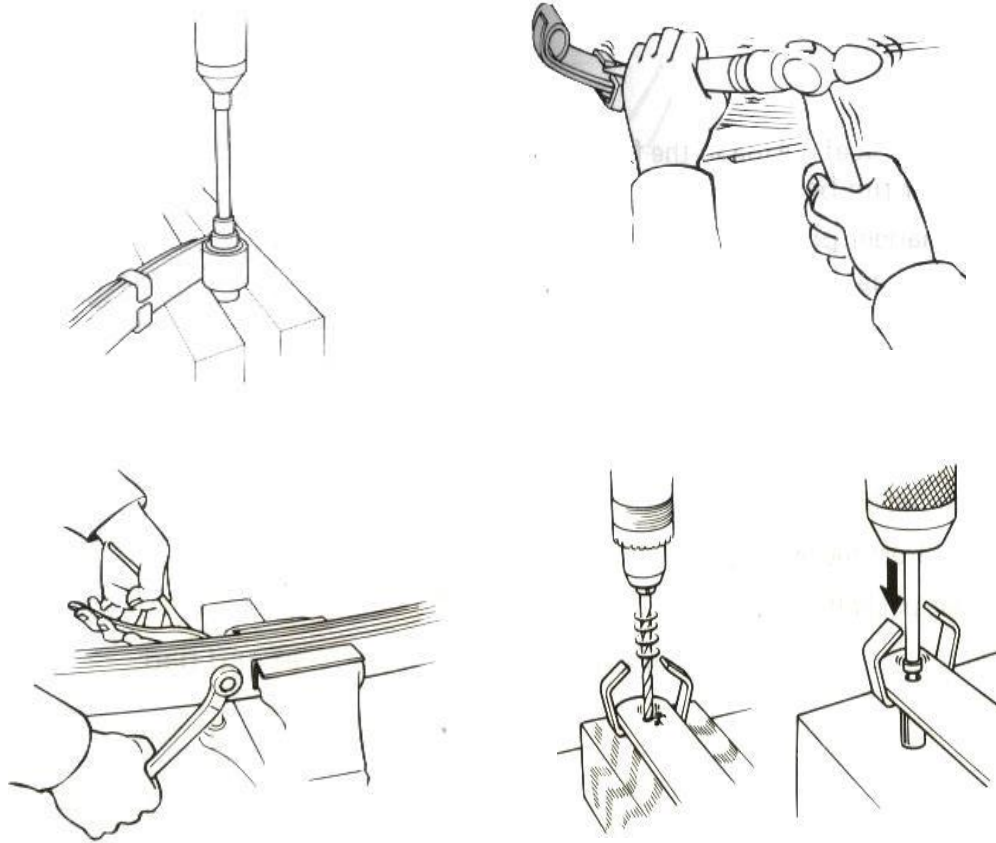
Hình 1.25 Tháo rời bộ nhíp
