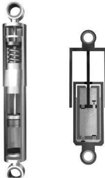
Hình 1.16. Giảm xóc ống loại 2 ống
