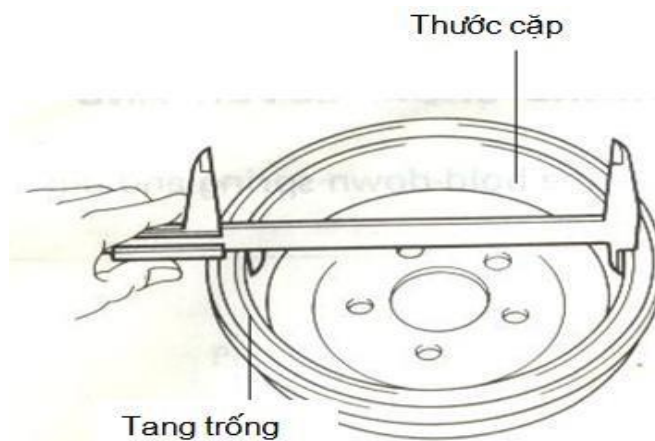
Hình 3.11 Kiểm tra tang trống phanh
