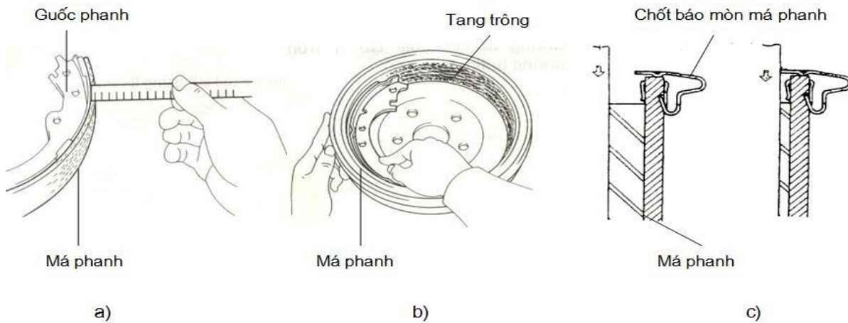
Hình 3.10 Kiểm tra cơ cấu phanh
