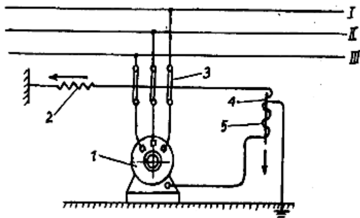
Hình 2-14 Cắt điện bảo vệ tự động
