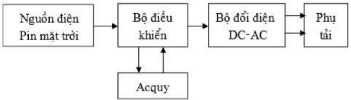
Hình 3.4: Sơ đồ khối hệ thống điện mặt trời Hệ
