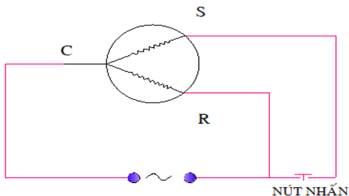
Hình 3.1: Sơ đồ khởi động động cơ tủ lạnh.
