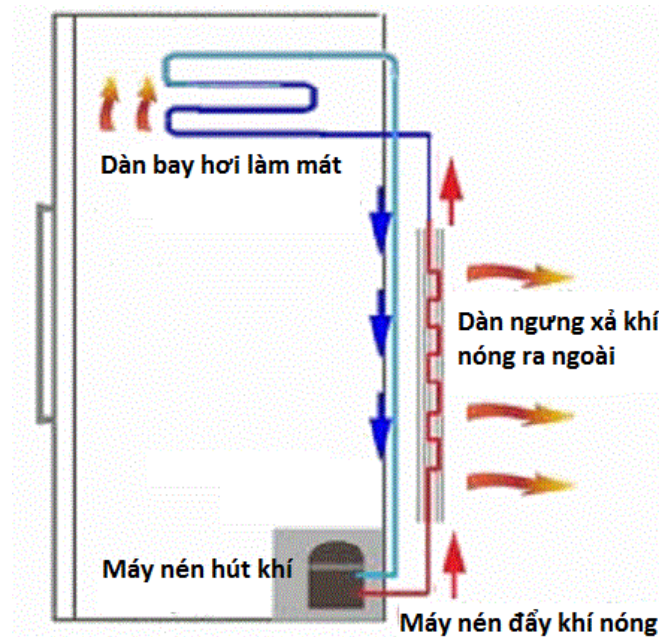
Hình 1.1: Sơ đồ nguyên lý tủ lạnh trực tiếp.
