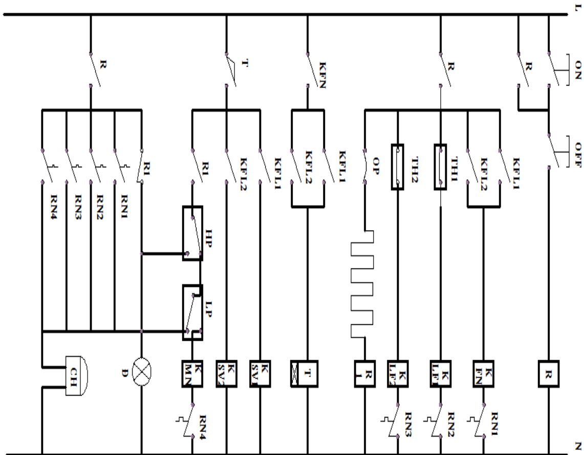
Hình 12.2: Bản vẽ thiết kế hệ thống lạnh.
