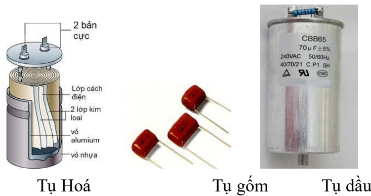
Hình 4.8: Các loại tụ điện.
