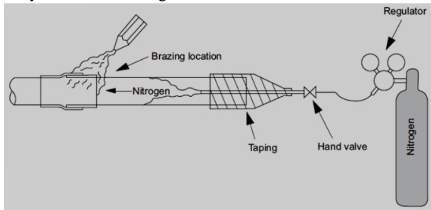
Hình 12.3: Hàn ống.
