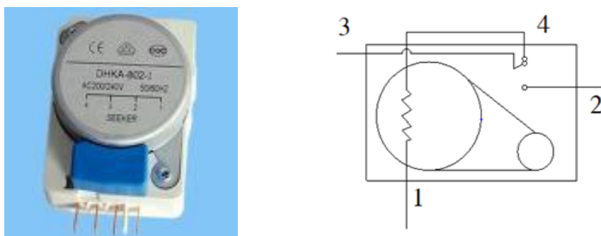
Hình 4.11: Cấu tạo timer loại 2.
