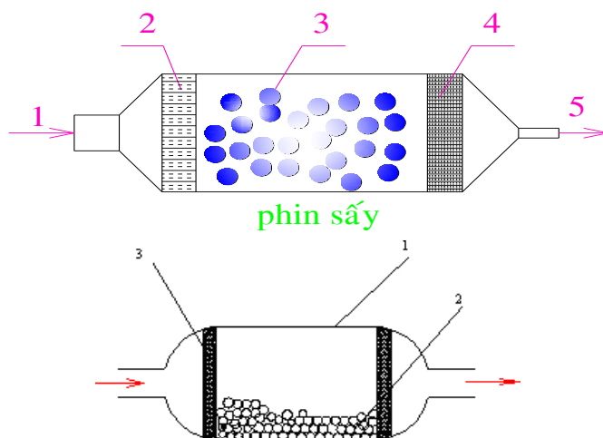
Hình 1.10: Phin sấy lọc nước cho máy lạnh freon cỡ nhỏ và cỡ nhỏ.
