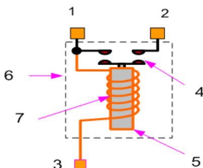
Hình 4.4: Cấu tạo Rơ le khởi động.
