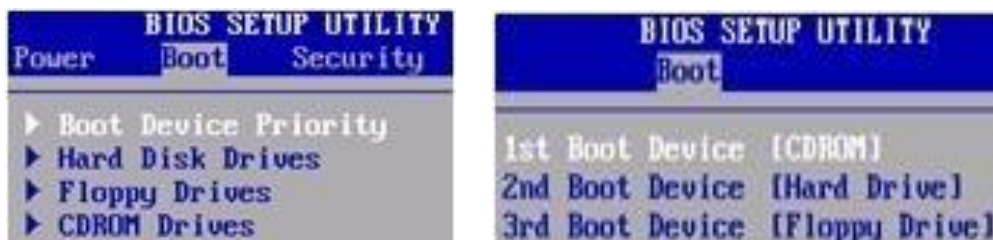
Hình 3.14: Chọn thứ tự boot ổ đĩa
