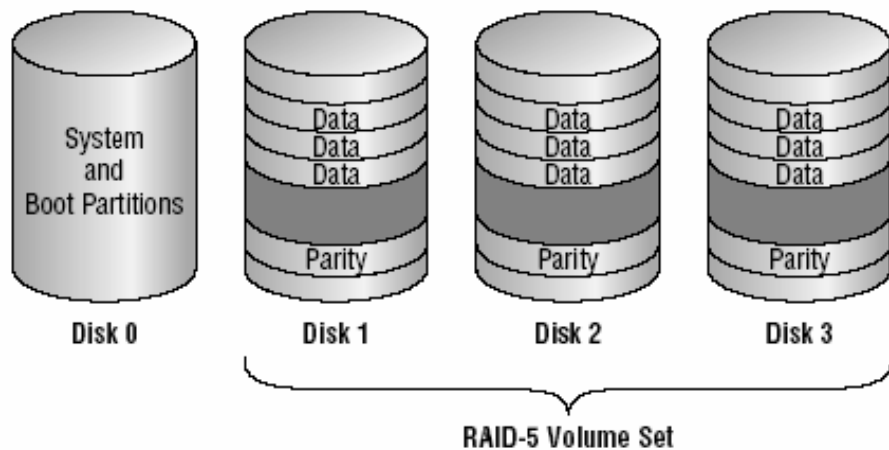
Hình 5.5: Volume RAID-5
