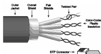
Hình 3.7– Mô tả cáp STP.
