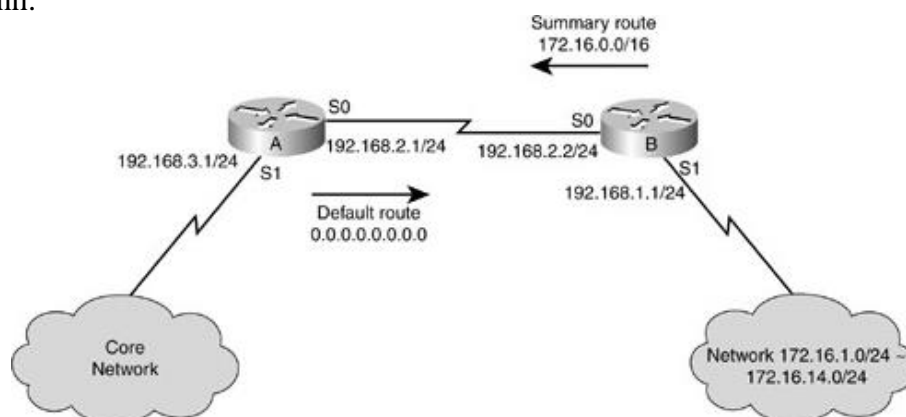
Hình 6.30 Mô hình EIGRP
