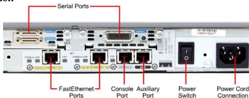
Hình 4.1 Các cổng kết nối của Router
