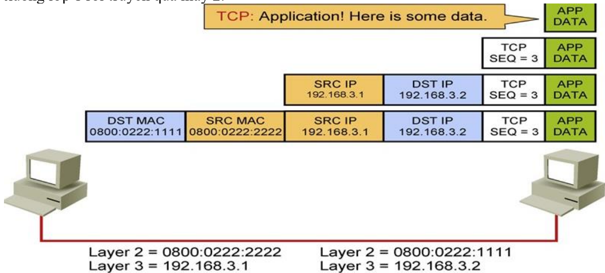
Hình 4.21 Minh họa quá trình trao đổi gói tin giữa hai máy trong mạng Máy 2 nhận được chuyển thành frame, gỡ bỏ các header ở các lớp 2, 3, 4... và trả về data cho Application.
