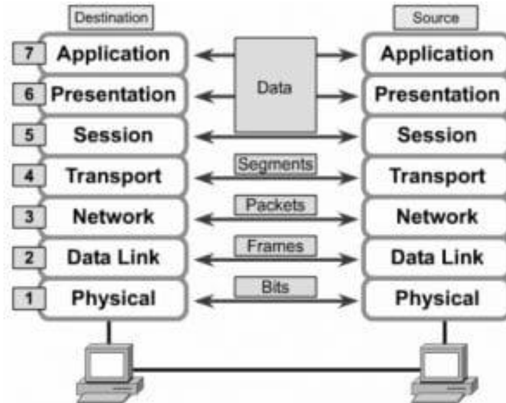
Hình 3.10 Data, Segments, Packets, Frames, Bits trong mô hình OSI
