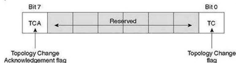
Hình 6.19: trường cờ trong BPDU cấu hình
