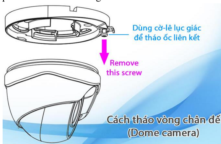
Hình 2.22 Cách tháo vòng chân đế camera dome để gắn lên trần nhà
