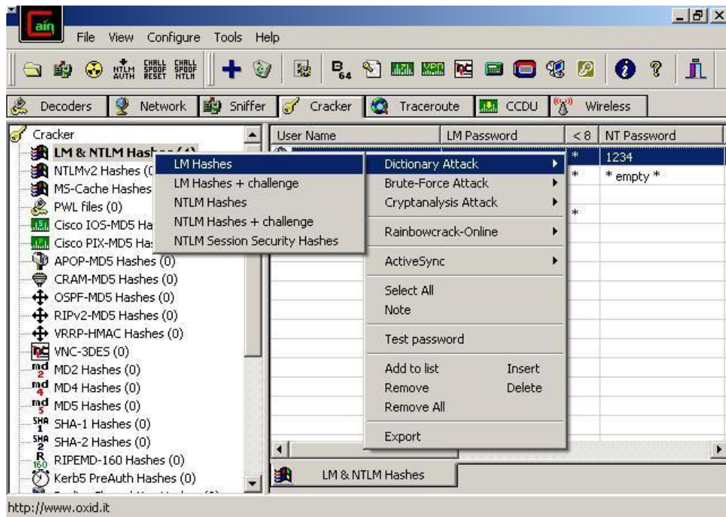
Hình 1.8 Chạy chương trình Cain & Abel
