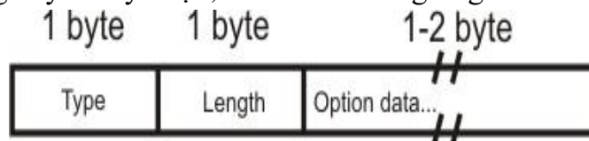
Hình 2.8 Gói TCP
