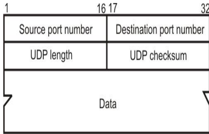
Hình 2.4 Cấu trúc gói tin
