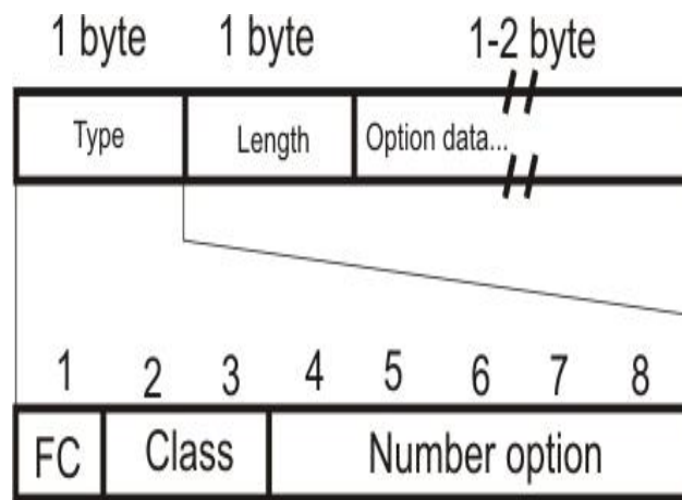
Hình 2.3 Cấu trúc của gói tin
