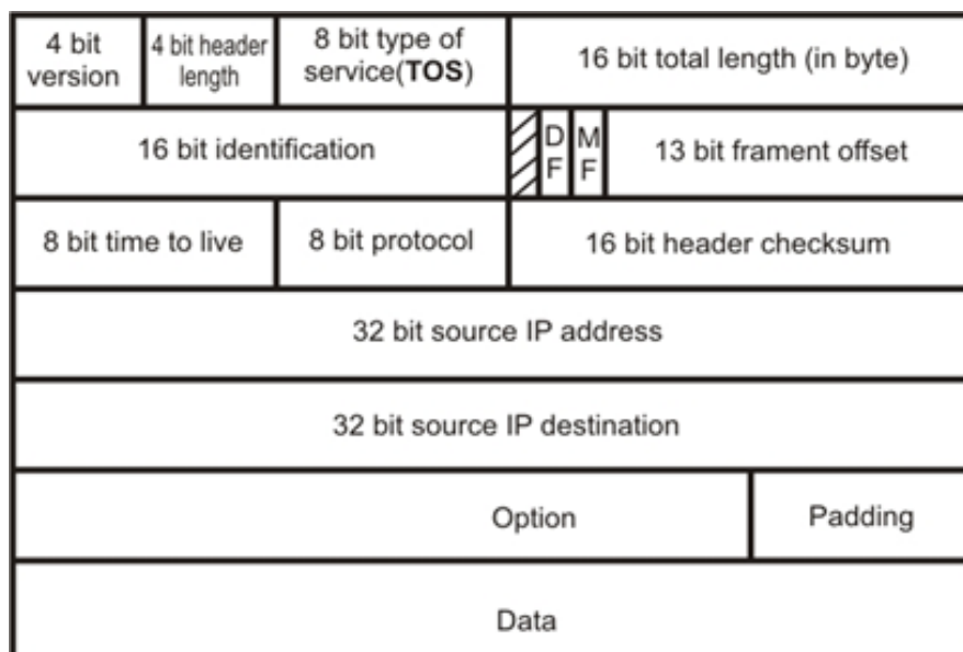
Hình 2.1 Cấu trúc của gói IP
