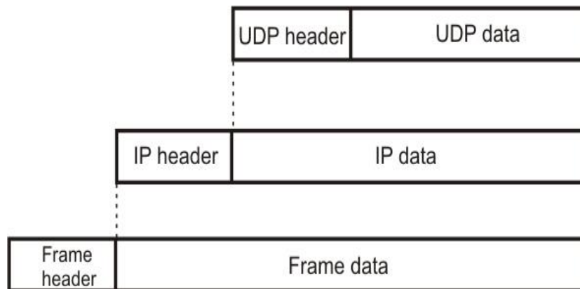
Hình 2.5: quá trình đóng gói UDP
