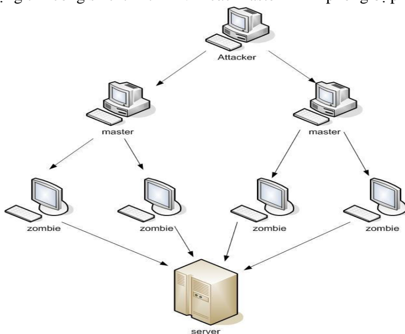
Hình 1.2 Minh họa tấn công DDOS
