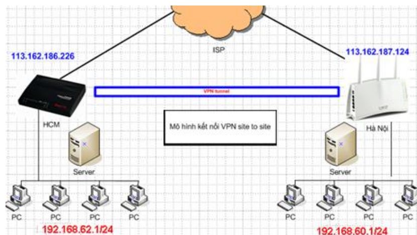
Hình 3.15 Mô hình kết nối
