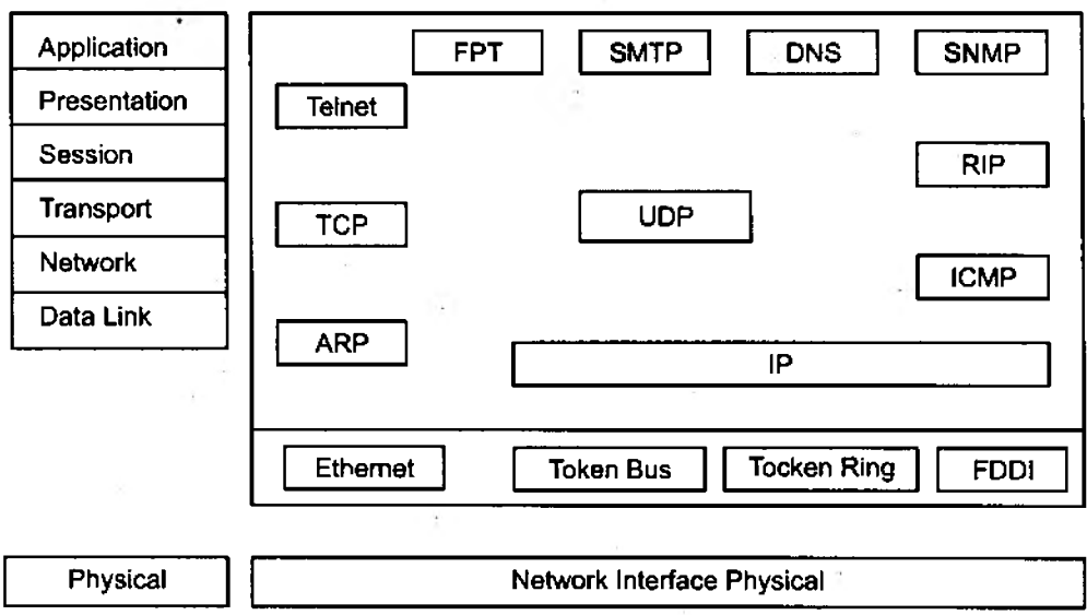
Hình 2.3. Mô hình, TCP/IP và các ứng dụng
