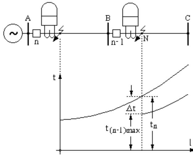
Hình 2.6 : Phối hợp các đặc tính của bảo vệ dòng cực đại có đặc tính thời gian phụ thuộc giới hạn. N : Điểm ngắn mạch tính toán
