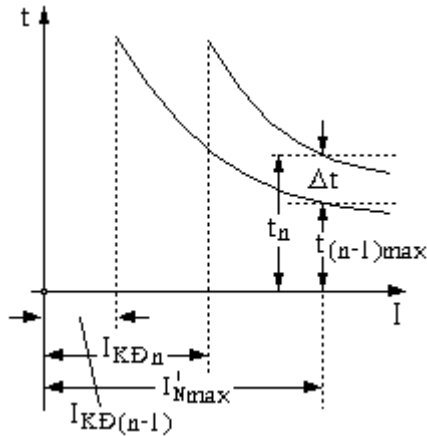
Hình 2.7 : Phối hợp đặc tính thời gian làm việc phụ thuộc có giới hạn của các bảo vệ dòng cực đại trong hệ tọa độ dòng - thời gian.
