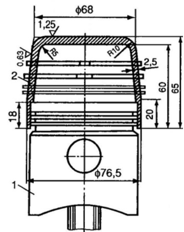
Hình 7.10 Chụm lắp séc măng 1-piston; 2-chụm lắp séc măng
