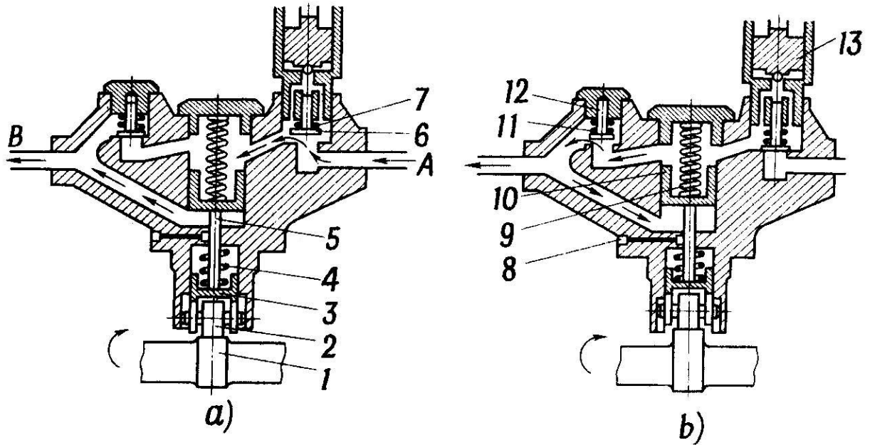
Hình 9.11. Bom chuyển nhiên liệu
