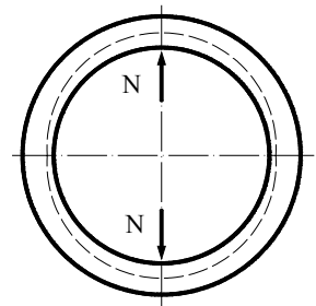
Hình 1.16. Dạng hao mòn hướng kính của xi lanh
