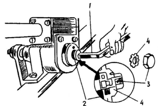
Hình 10.30. Điều chỉnh khe hở ăn khớp của trục vít-con lăn. 1-clê. 2-đai ốc điều chỉnh. 3-ốc hãm. 4-đệm hãm
