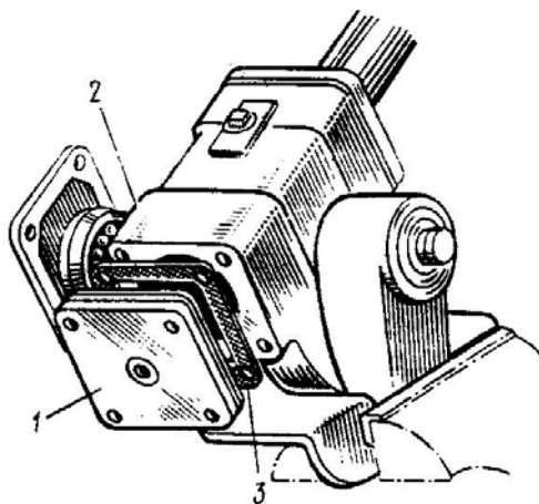
Hình 10.29. Điều chỉnh khe hở chiều trục cơ cấu lái kiểu trục vít con lăn 1-Nắp. 2-Các te cơ cấu lái. 3-Đệm điều chỉnh
