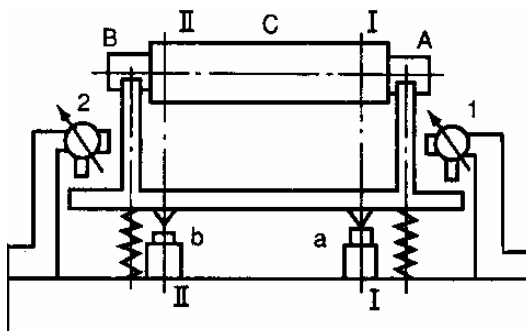
Hình 6.27 Nguyên lý thiết bị cân bằng trên 2 mặt phẳng chọn trước 1,2_ cảm biến biên độ dao động khung a,b_ các ổ tì; A,B_ các ổ đỡ trục trục trên khung dao động.
