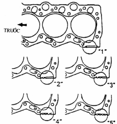
Hình 7.13 Khắc chỉ thị độ dày đệm nắp
