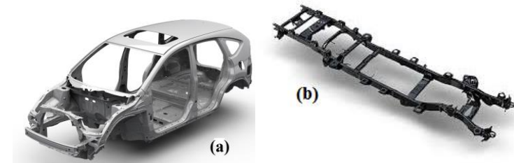
Hình 3-11: Khung xe
