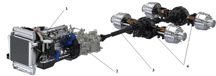
Hình 3-1đ: Hệ thống truyền lực trên xe tải cỡ lớn hai cầu sau chủ động
