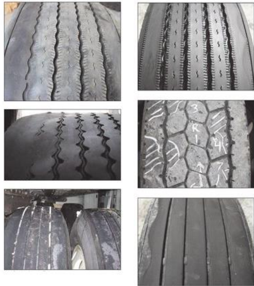
Hình 8.7: các dạng mòn lốp không đều
