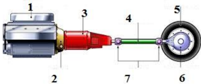
Hình 3-1a: Sơ đồ bố trí hệ thống truyền lực ô tô 1-Động cơ, 2-Ly hợp, 3-Hộp số, 4-các đặng, 5-bánh xe, 6-cầu chủ động, 7-khớp các đặng.
