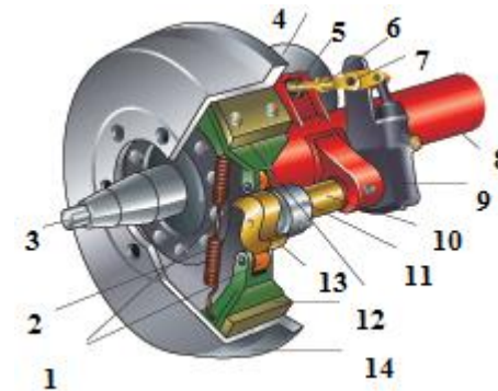
Hình 3-27: Cơ cấu phanh của hệ thống phanh dẫn động khí nén 1-con lặn; 2-lò xo hồi vị; 3-trục; 4-bầu phanh; 5-thanh đẩy; 6-ê cu điều chỉnh hành trình thanh đẩy; 7-khớp quay; 8-câu; 10-trục cam; 12-má phanh; 13-cam.
