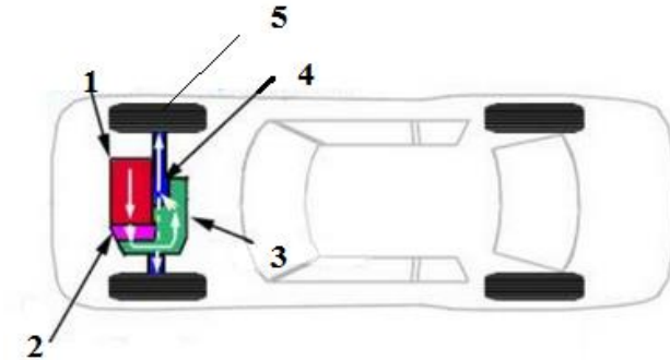
Hình 3- 1 Hệ thống truyền lực ô tô con có cầu trước chủ động 1- Động cơ, 2-Ly hợp, 3-Hộp số, 4-các đặng, 5-bánh xe chủ động
