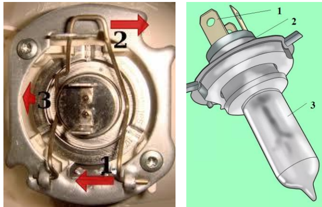
Hình 8.21: Đèn pha
