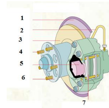
Hình 3-25: cơ cấu phanh đĩa 1-vỏ chắn bụi; 2-ống dầu; 3-đĩa phanh; 4-bu lông lắp bánh xe; 5-xy lanh phanh; 6-bích lắp bánh xe; 7-má phanh.
