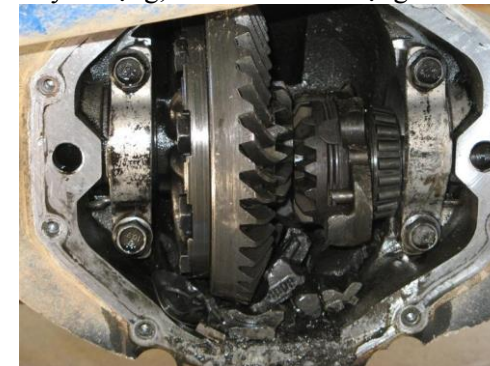
Hình 6.14: bộ vi sai của cầu chủ động bị hỏng
