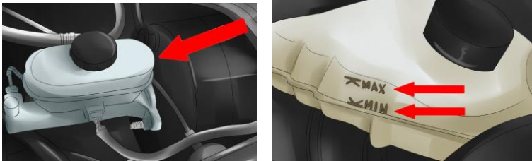
Hình 6.11: Kiểm tra, bổ sung dầu ly hợp
