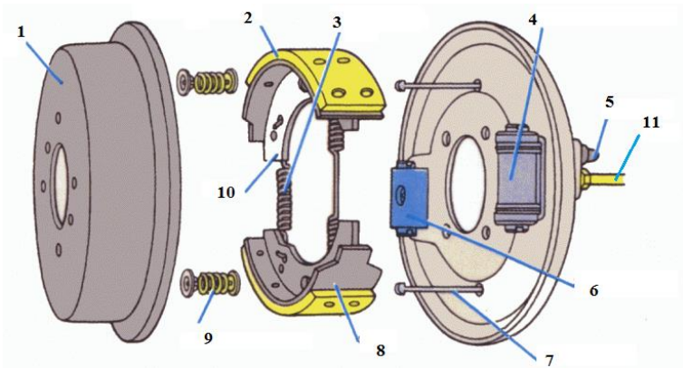
Hình 3-26: Cơ cấu phanh tang trống 1-Trống phanh; 2- má phanh; 3-lò xo hồi vị; 4-xy lanh phanh bánh xe; 5-nút xả air; 6-tự guốc phanh; 7-chốt hãm; 8,10-guốc phanh, 11 đường dầu phanh.
