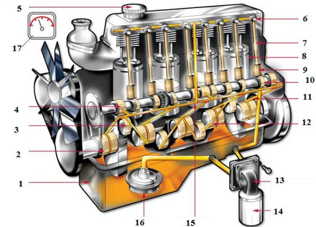
Hình 2-5: Hệ thống bôi trơn động cơ 1-các te chứa dầu, 2-bạc đầu trục khuỷu, 3-bạc bánh răng trung gian, 4-bạc trục cam, 5-Nắp đổ dầu, 6-cò cam, 7-đũa đẩy, 8- xylanh, 9-con đội, 10-cam, 11-bạc biên, 12-bạc trục khuỷu, 13-bơm dầu, 14-lọc dầu, 15-ống dẫn dầu chính, 16-phao hút dầu, 17-đồng hồ báo áp suất dầu.
