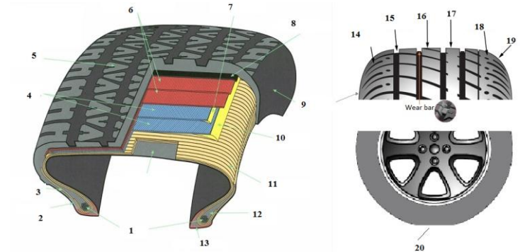
Hình 2-14 Lốp 1-Sợi thép tanh lốp; 2- vùng tanh lốp; 3-lốp sợi bố; 4-lốp màng bố thép, 5-gai lốp, 6-lốp bó đệm ni lon, 7-Nệm đai bố; 8-lốp cao su đệm; 9-thành lốp; 10-lốp nệm vai lốp; 11- Lốp bó nilon lốp (vỏ); 12-đỉnh thành lốp; 13-chân tan lốp; 14-gai thành lốp; 15-rãnh thoát nước; 16-gai tạo ma sát; 17-rãnh định hướng; 18- Rãnh ; 19-Gai vai lốp.
