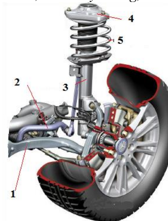
(c) Hệ thống treo độc lập MC Pherson
