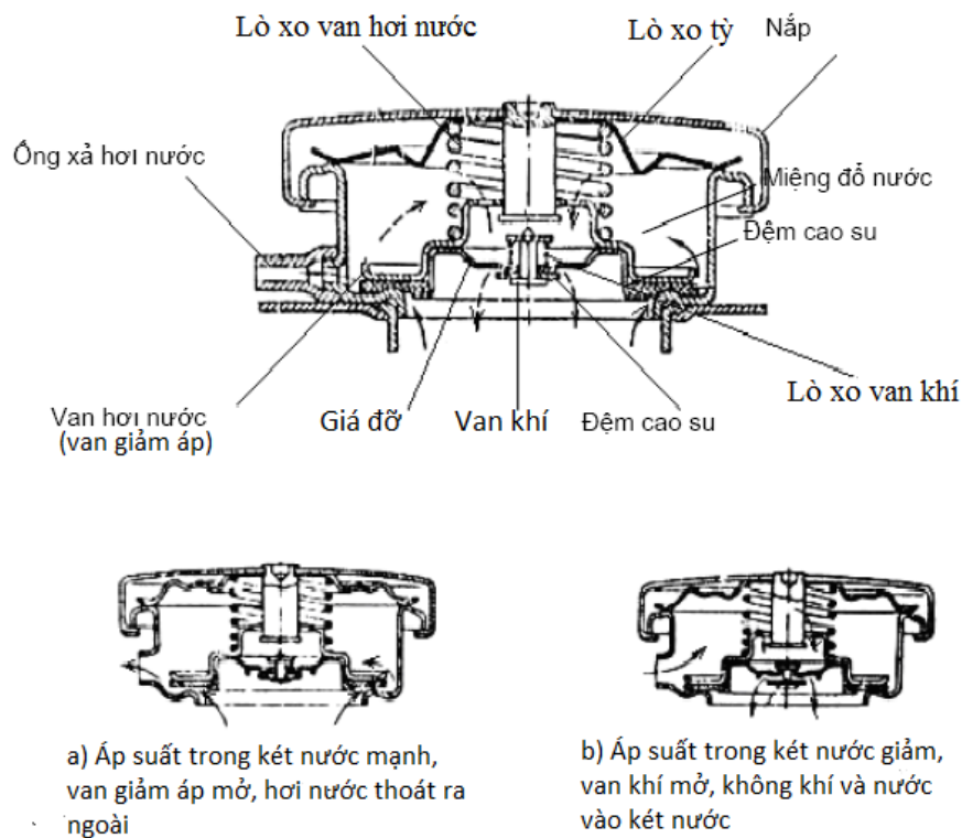
Hình 4.16. Cấu tạo, nguyên lý hoạt động của nắp két nước
