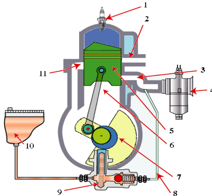
Hình 1.2. Bôi trơn bằng dầu pha trong nhiên liệu
