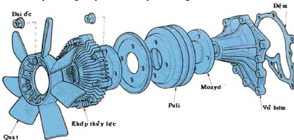
Hình 4.11. Dẫn động quạt gió bằng thủy lực
