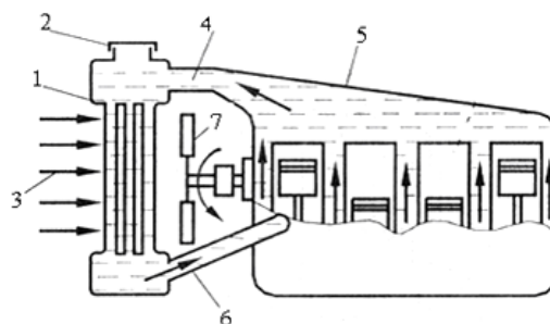
Hình 4.5. Làm mát bằng nước kiểu đối lưu tự nhiên
