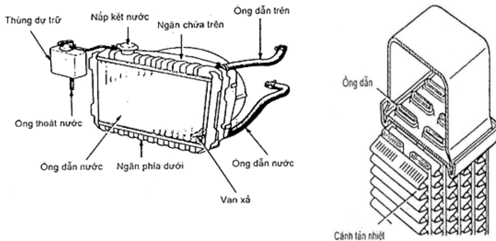
Hình 4.15. Cấu tạo két nước
