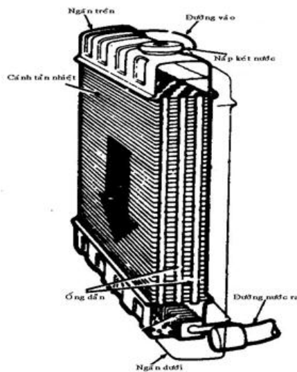
Hình 4.14. Kết nước làm mát
