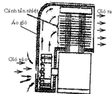
Hình 4.2. Hệ thống làm mát bằng gió cưỡng bức
