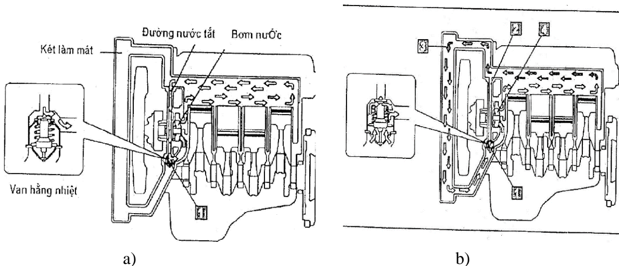
Hình 4.22. Bố trí đường nước vào
