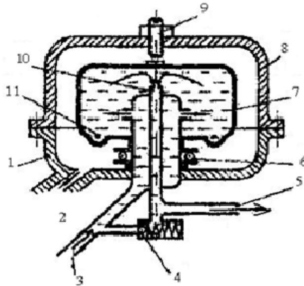
Hình 1.15. Bầu lọc li tâm
