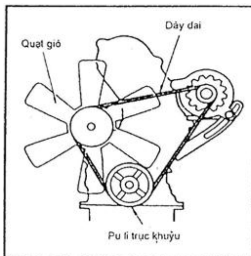
Hình 4.12. Dẫn động bằng cơ khí
