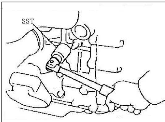
Hình 2.2. Kiểm tra áp suất nhớt
