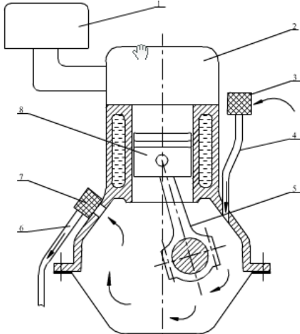
Hình 1.18. Thông hơi động cơ Diesel 1. Lọc gió, 2. Nắp máy, 3. Lọc khí thông gió, 4. Ống gió vào, 5. Thanh truyền, 6. Ống gió ra, 7. Lọc ngăn dầu, 8. Pít tông
