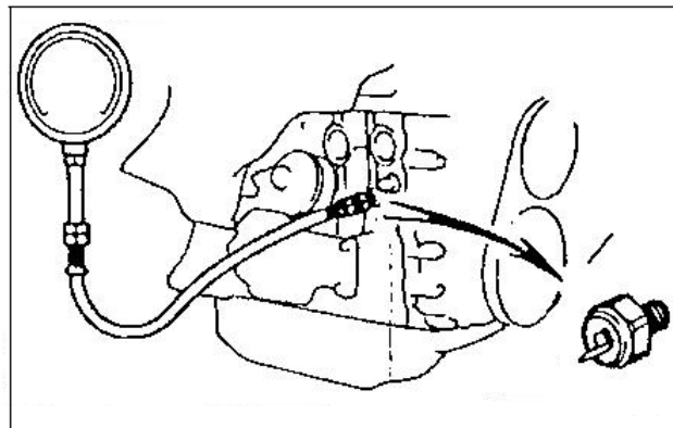
Hình 2.2. Kiểm tra áp suất nhớt
