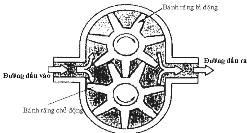
Hình 1.8. Bơm bánh răng ăn khớp ngoài
