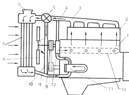
Hình 4.6. Sơ đồ hệ thống làm mát tuần hoàn cưỡng bức một vòng kín
