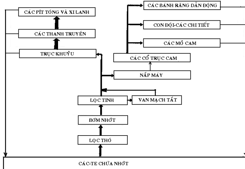
Hình 1.6. Sơ đồ hệ thống bôi trơn
