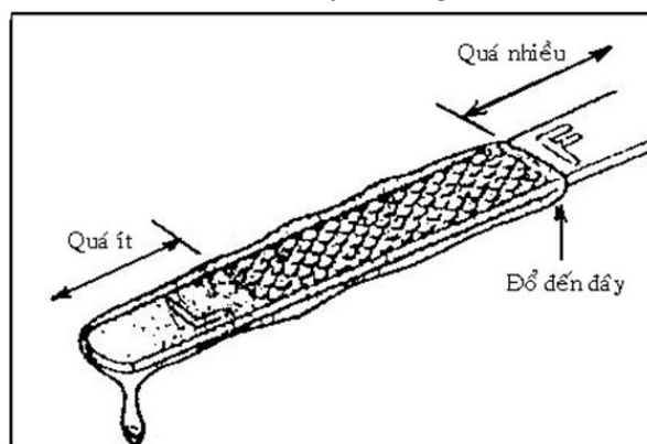
Hình 2.1 . Kiểm tra mức dầu bôi trơn
