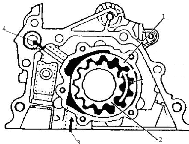
Hình 1.7. Bơm bánh răng ăn khớp trong
