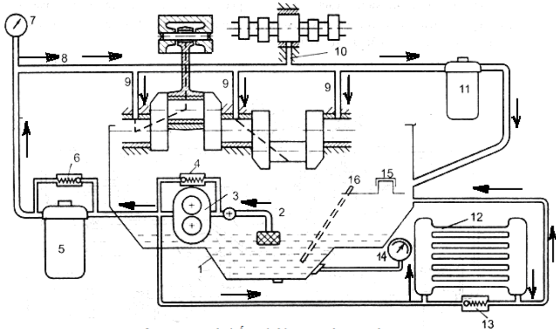
Hình 1.3. Hệ thống bôi trơn các te ướt
