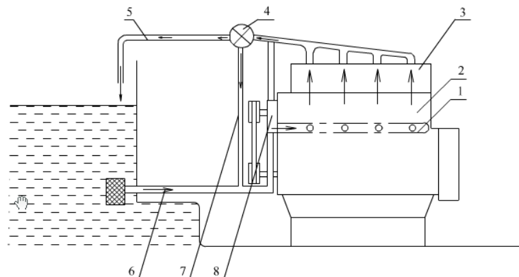
Hình 4.7. Sơ đồ hệ thống làm mát tuần hoàn cưỡng bức một vòng hở
