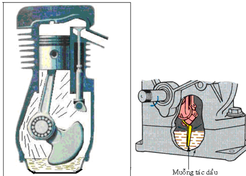
Hình 1.1. Bôi trơn bằng muông tác dầu (bôi trơn bằng vùng tóa)
