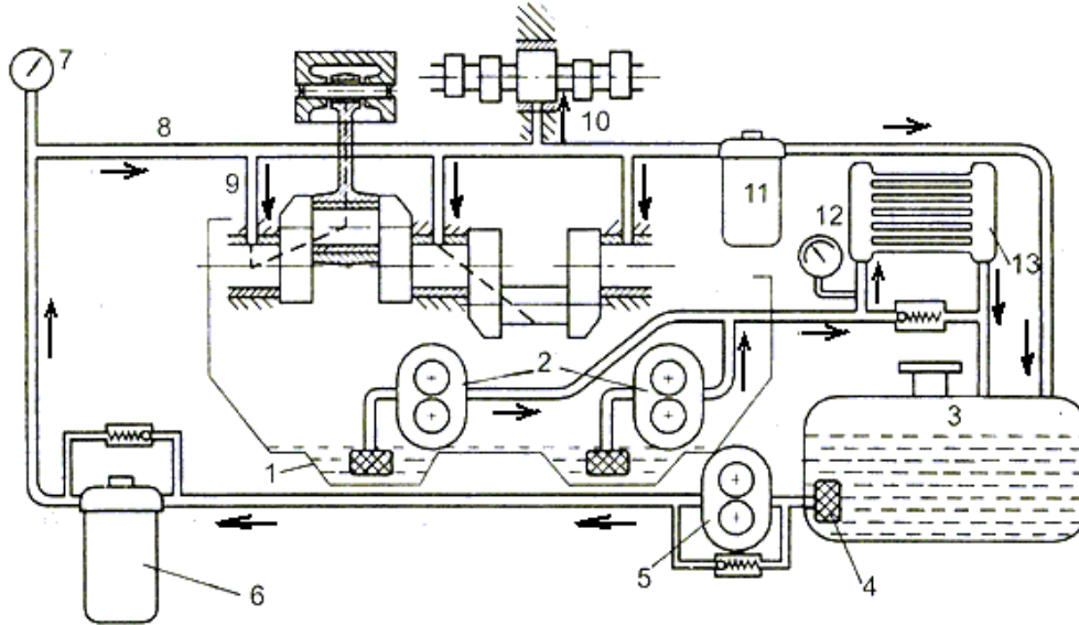
Hình 1.4. Hệ thống bôi trơn các te khô
