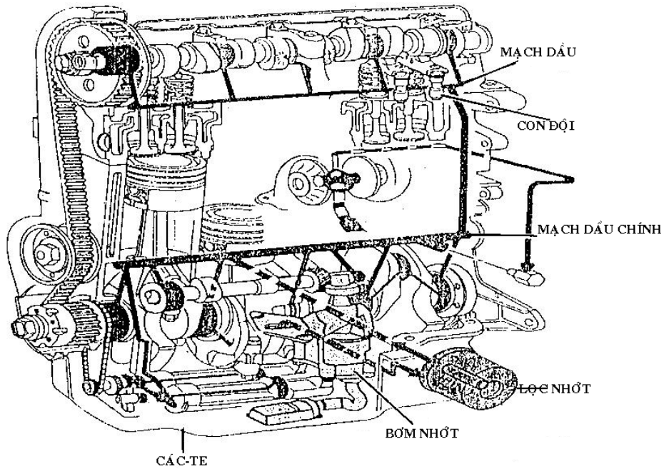
Hình 1.5. Sơ đồ mạch dầu bôi trơn động cơ
