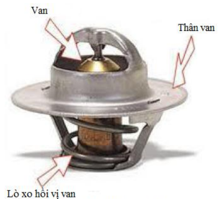
Hình 4.19. Van hằng nhiệt
