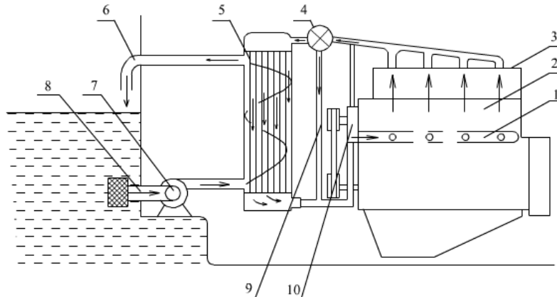
Hình 4.6. Hệ thống làm mát tuần hoàn cưỡng bức kiểu hai vòng 1. đường nước phân phối; 2. Thân máy; 3. Nắp xy lanh; 4. Van hằng nhiệt; 5. Két làm mát; 6. Đường nước ra vòng hở; 7. Bơm nước vòng hở; 8. Đường nước vào vòng hở; 9. Đường nước tắt về bơm vòng kín; 10. Bơm nước vòng kín.
