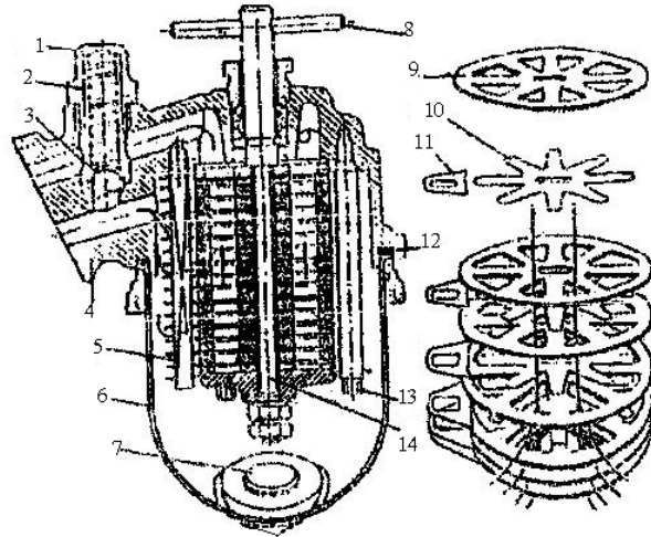
Hình 1.13. Kết cấu bầu lọc thô
