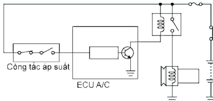
2.37. Mạch điện công tắc áp suất
