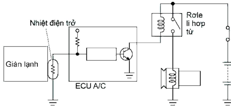
2.43. Điều khiển nhiệt độ giàn lạnh
