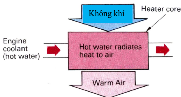
Hình 2.1. Nguyên lý bộ sưởi dùng nước làm mát động cơ
