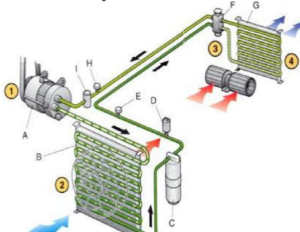
1.16. Sơ đồ thiết bị hệ thống
