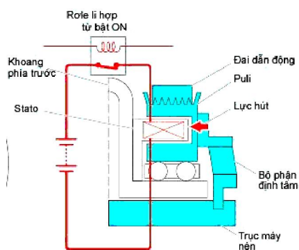
2.18. Cấp điện cho li hợp
