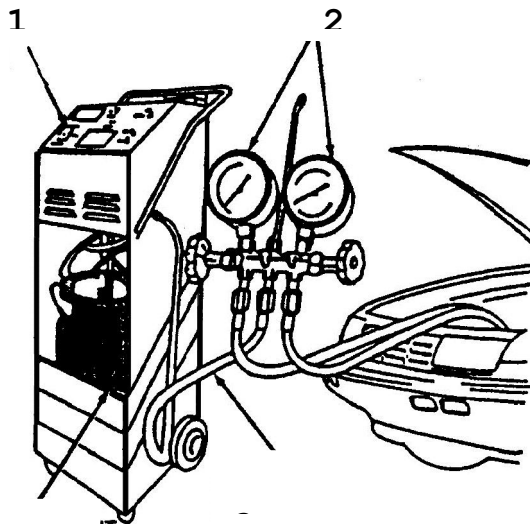
Hình 4.4. Trạm thiết bị dùng để thu hồi khí xả và thu hồi lại môi chất lạnh :
