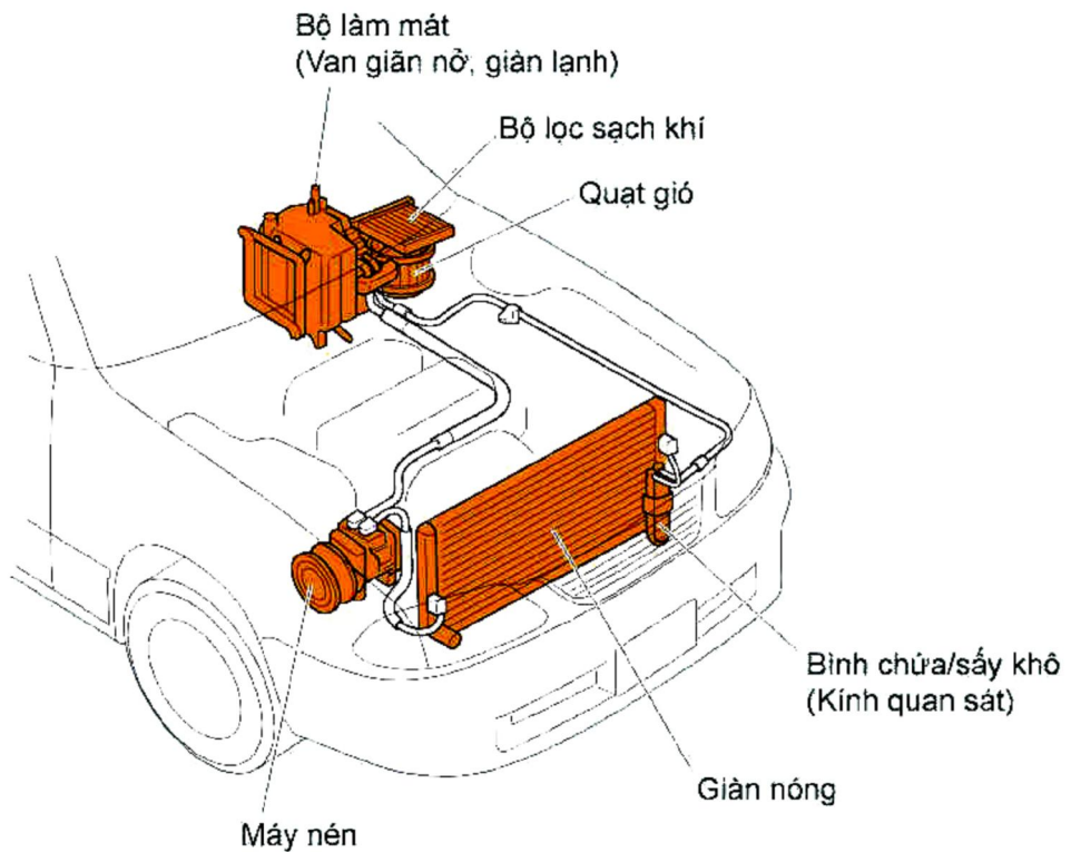
1.17. Sơ đồ chu trình làm lạnh khép kín
