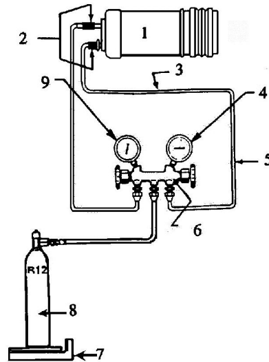
Hình 4.11. Lắp ráp thiết bị để nạp ga từ bình chứa môi chất lạnh loại lớn:
