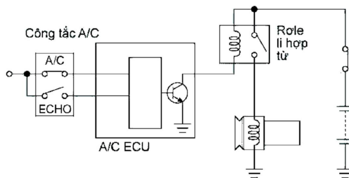
2.47. Hệ thống điều khiển máy nén 2 giai đoạn
