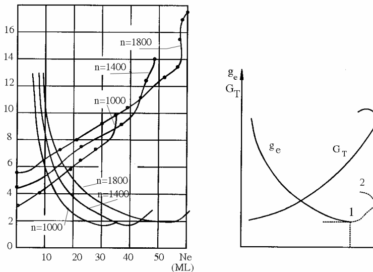
a) Động cơ cácbarato; b) Động cơ diesel.
