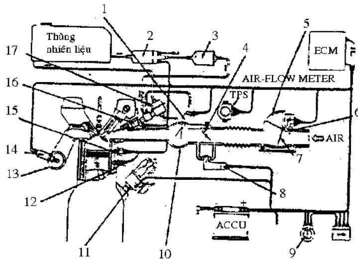
Hình 3- 21. Hệ thống phun nhiên liệu điện tử Bosh L dùng van bướm để đo lưu lượng không khí
