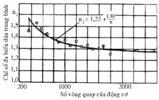
Hình 7-6. thị chỉ thị cơ có bộ khí 4 kỳ
