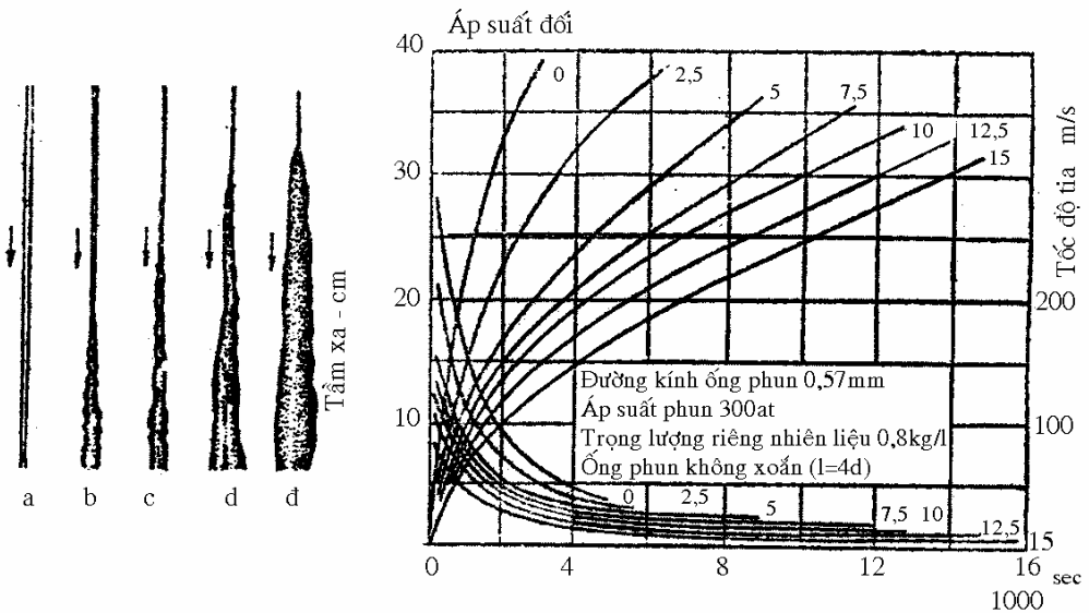
Hình 4-2. Ảnh chụp chùm hạt nhiên liệu với các áp suất chống đối khác nhau và sự biến thiên tâm xa của tia nhiên liệu
