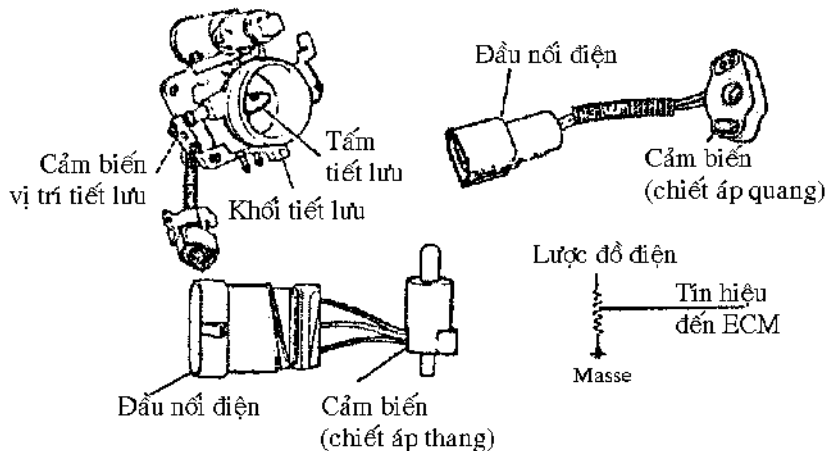
Hình 3-17. Sơ đồ mạch biến vị trí bướm xoay
