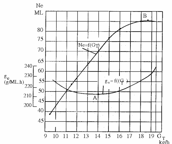
Hình 8-8. Đặc tính điều chỉnh theo lượng phun nhiên liệu
