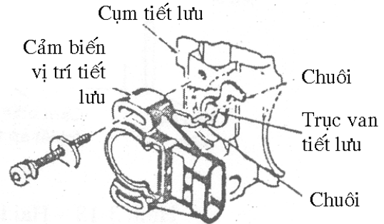
Hình 3-16. Vị trí của cảm biến vị trí tiết lưu trên khối tiết lưu
