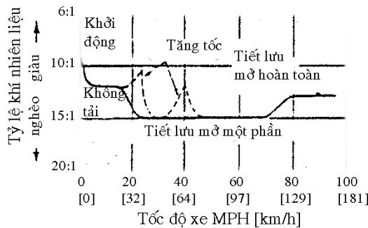
Hình 3-6. Bảng tỷ lệ nhiên liệu – khí tiêu biểu tương ứng với các điều kiện hoạt động của động cơ
