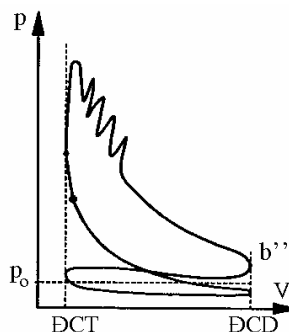
Hình 6-3. Đồ thị công cháy kích nổ
