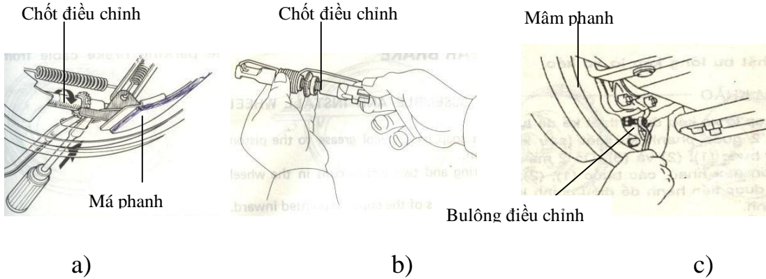
Hình 5 - 28. Kiểm tra và điều chỉnh khe hở cơ cấu phanh a) Xoay chốt điều chỉnh; b) Chốt điều chỉnh c) Điều chỉnh bulông cam lệch tâm
