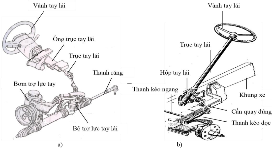
Hình 5-19: Sơ đồ cấu tạo chung hệ thống lái ô tô
