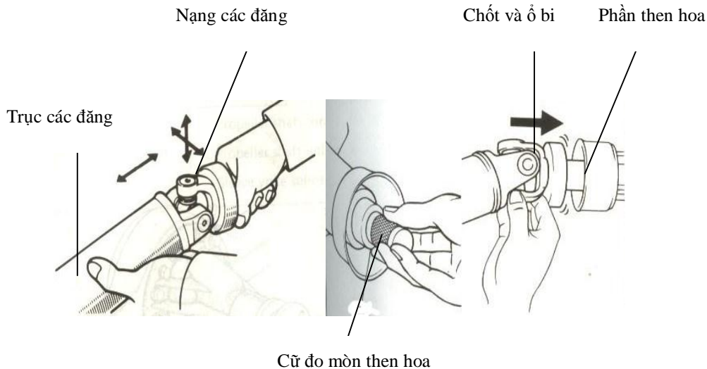
Hình 5 -3. Kiểm tra truyền động các đặng
