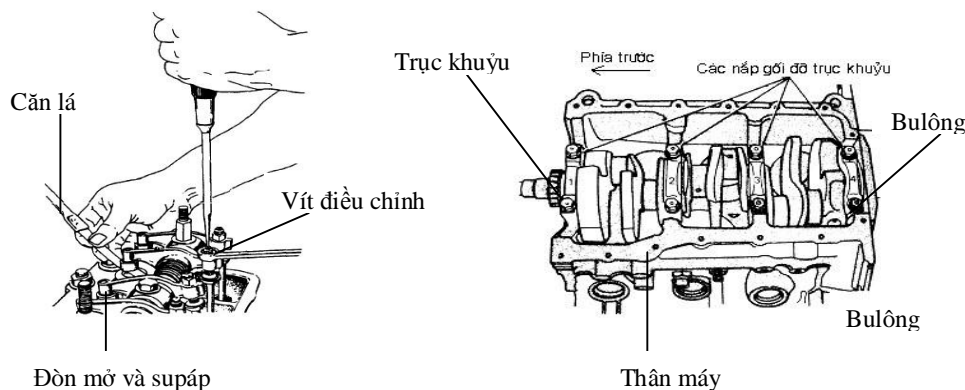
Hình 1- 4: Kiểm tra, điều chỉnh khe hở nhiệt và bạc lót, trực khuỷu a- Kiểm tra, điều chỉnh khe hở nhiệt b- Kiểm tra bạc lót, trực khuỷu
