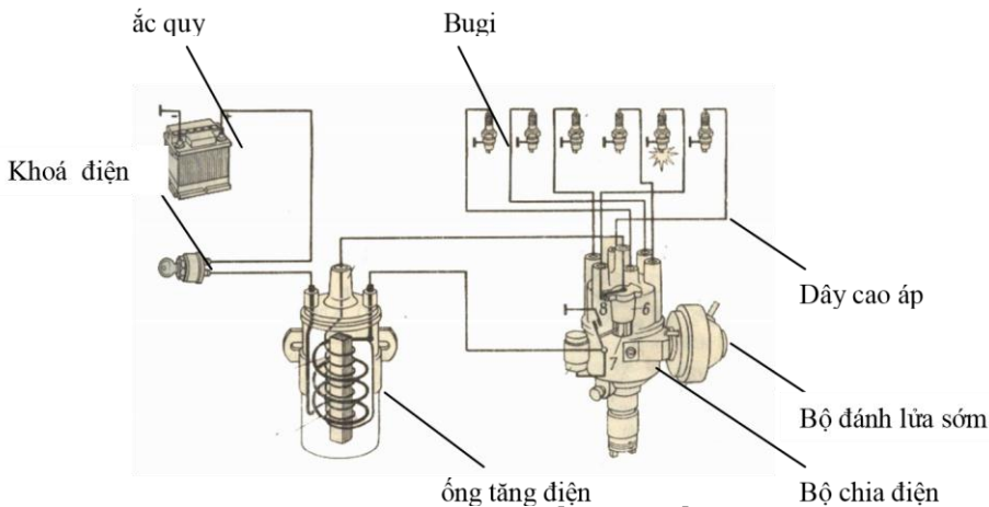
Hình. 13: Sơ đồ hệ thống đánh lửa trên ô tô
