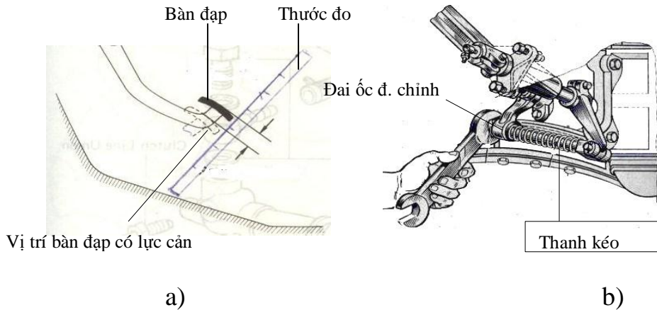
Hình 5-8. Kiểm tra và điều chỉnh hành trình tự do của bàn đạp ly hợp a. Kiểm tra; b. Điều chỉnh
