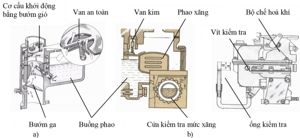
Hình 1.6. Kiểm tra mức xăng trong buồng phao
