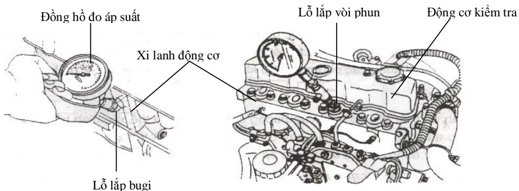
Hình 1.7: Kiểm tra áp suất nén của xi lanh
