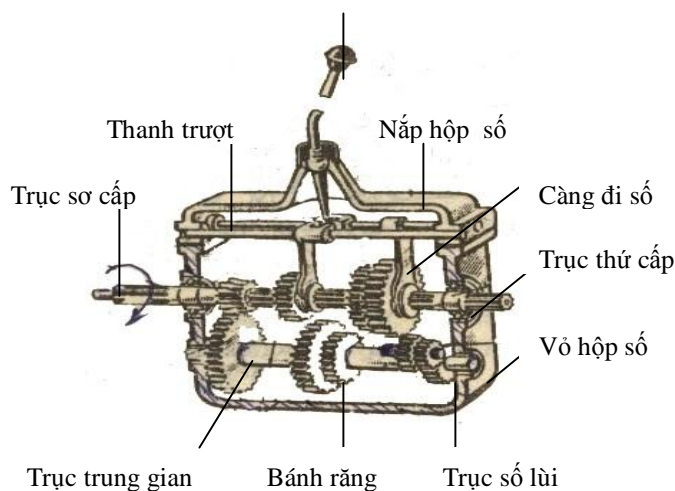
Hình 5-2: Cấu tạo hộp số cơ khí
