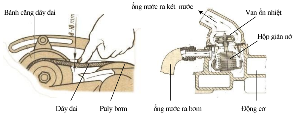
Hình 1.5: Kiểm tra độ căng dây đai và van ổn nhiệt
