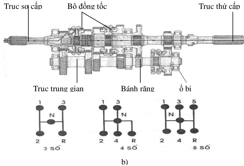
Hình 5-11. Cấu tạo hộp số cơ khí và các vị trí sang số a) Cấu tạo hộp số; b) Các vị trí đi số .
