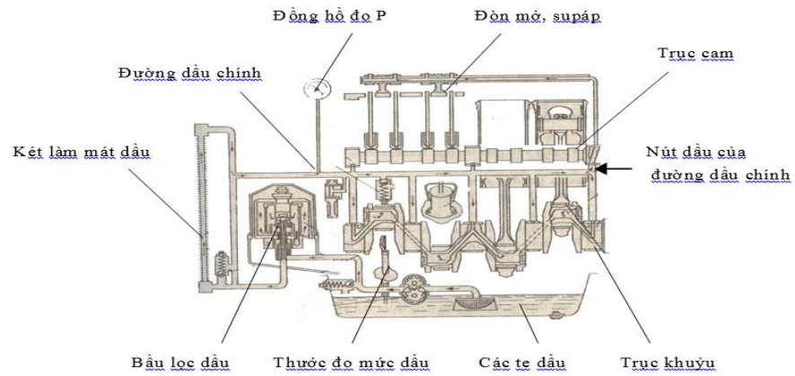
Hình 1.9: Kiểm tra áp suất đường dầu chính
