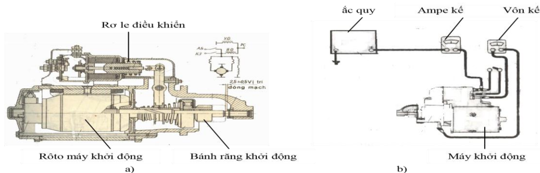
Hình. 1-2: Sơ đồ kiểm tra máy khởi động
