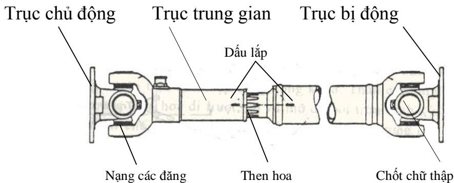
Hình 5 -12. Cấu tạo các đăng kép (đồng tốc)
