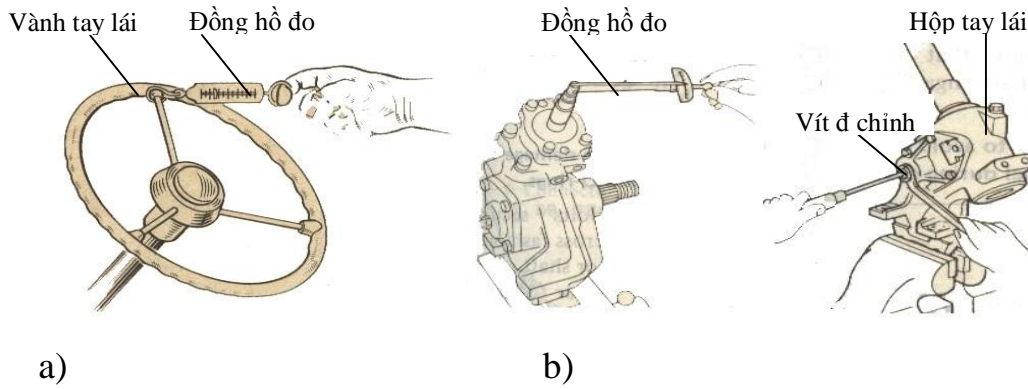
Hình 5 - 23. Kiểm tra và điều chỉnh lực quay vành tay lái
