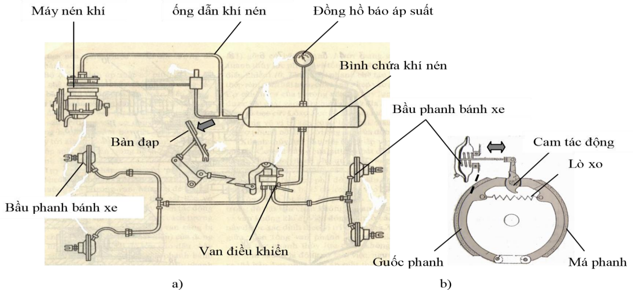
Hình 5-25. Sơ đồ cấu tạo hệ thống phanh khí nén a) Cấu tạo dẫn động phanh; b) Cấu tạo cơ cấu phanh
