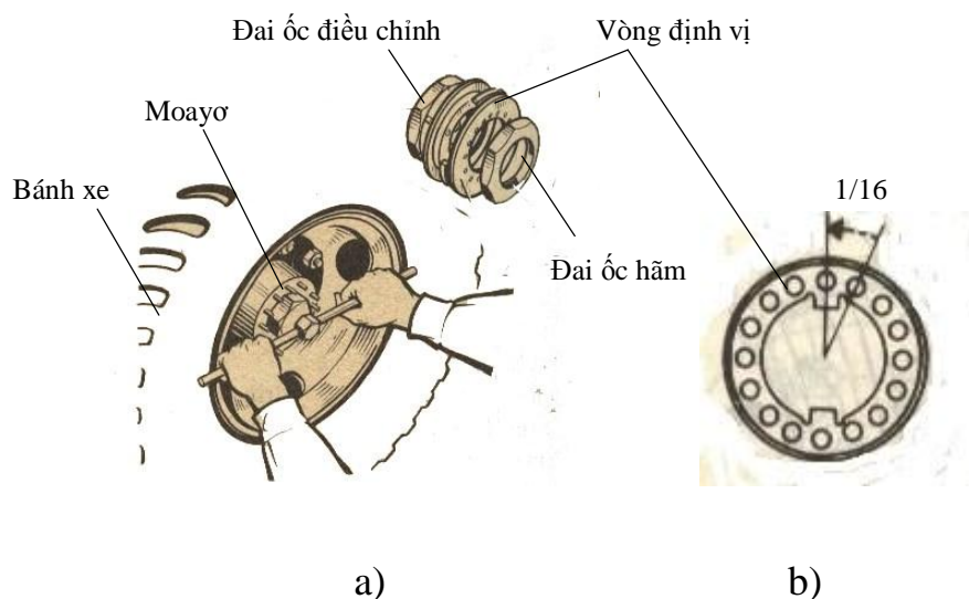
Hình 5 - 16. Kiểm tra và điều chỉnh độ rơ của moayơ bánh xe sau
