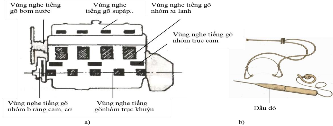
Hình 1-5. Các vùng nghe tiếng gõ động cơ và dụng cụ kiểm tra a) Sơ đồ các vùng nghe tiếng gõ b) Các dụng cụ kiểm tra tiếng gõ
