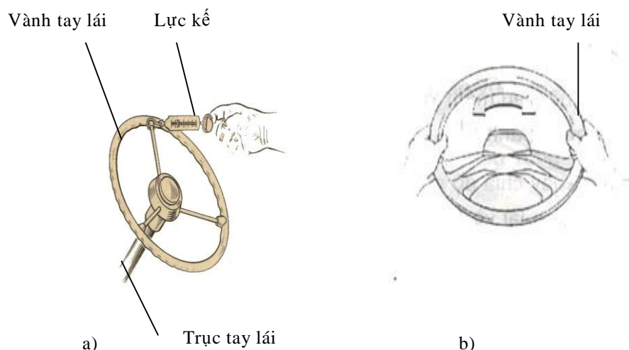
Hình. 5-6: Sơ đồ kiểm tra lực xoay vành tay lái
