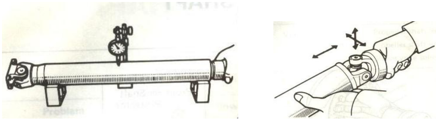
a- Kiểm tra trục cong b- Kiểm tra mòn chốt chữ thập và ổ bi Hình 5 -13. Kiểm tra truyền động các đăng
