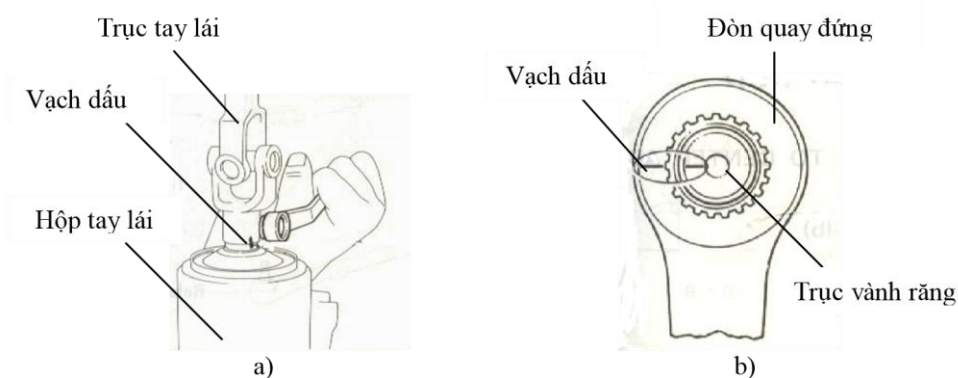
Hình 5 -20: Lắp đúng dấu các chi tiết của hệ thống lái ô tô
