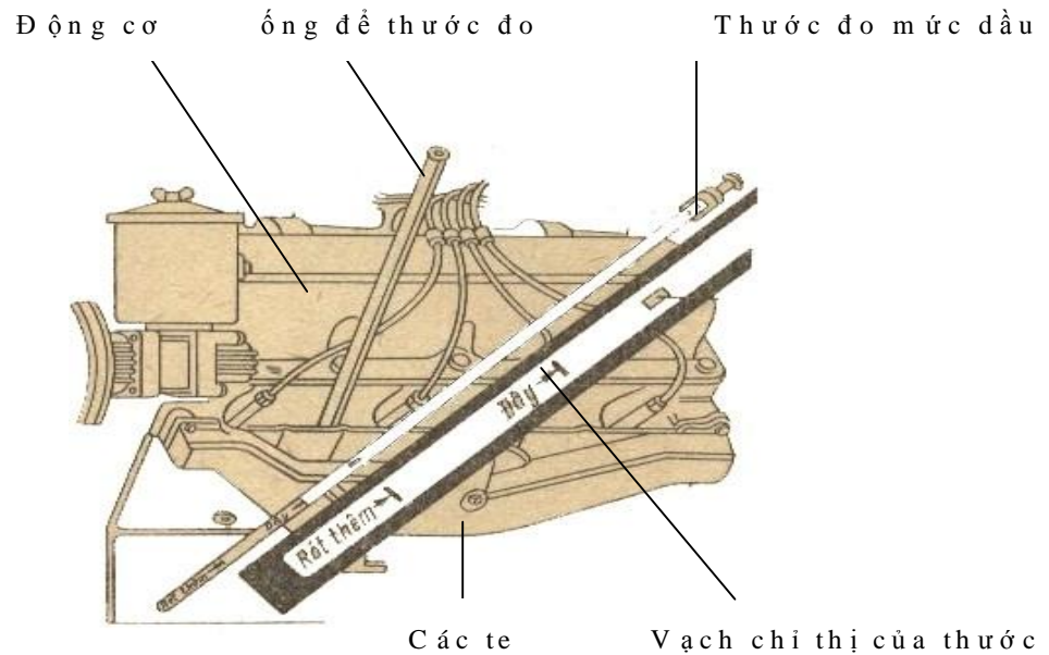
Hình 1.8: Kiểm tra mức dầu bôi trơn dầu bôi trơn
