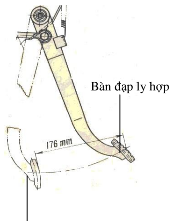
Hình. 5-9. Kiểm tra hành trình công tác của bàn đạp
