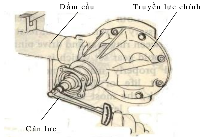
Hình 5 - 14. Kiểm tra và điều chỉnh
