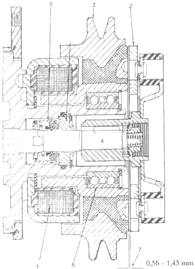
Hình 27. Kết cấu của bộ ly hợp điện từ trang bị trong buli máy nén : 1 Cuộn dây nam châm điện. 2. Đĩa bị động. 3. Bull. 4. Trục máy nén. 5 Vòng bị kẹp. 6. Phốt kim trực. 7. Khe hở khi bộ ly hợp cắt khớp.
