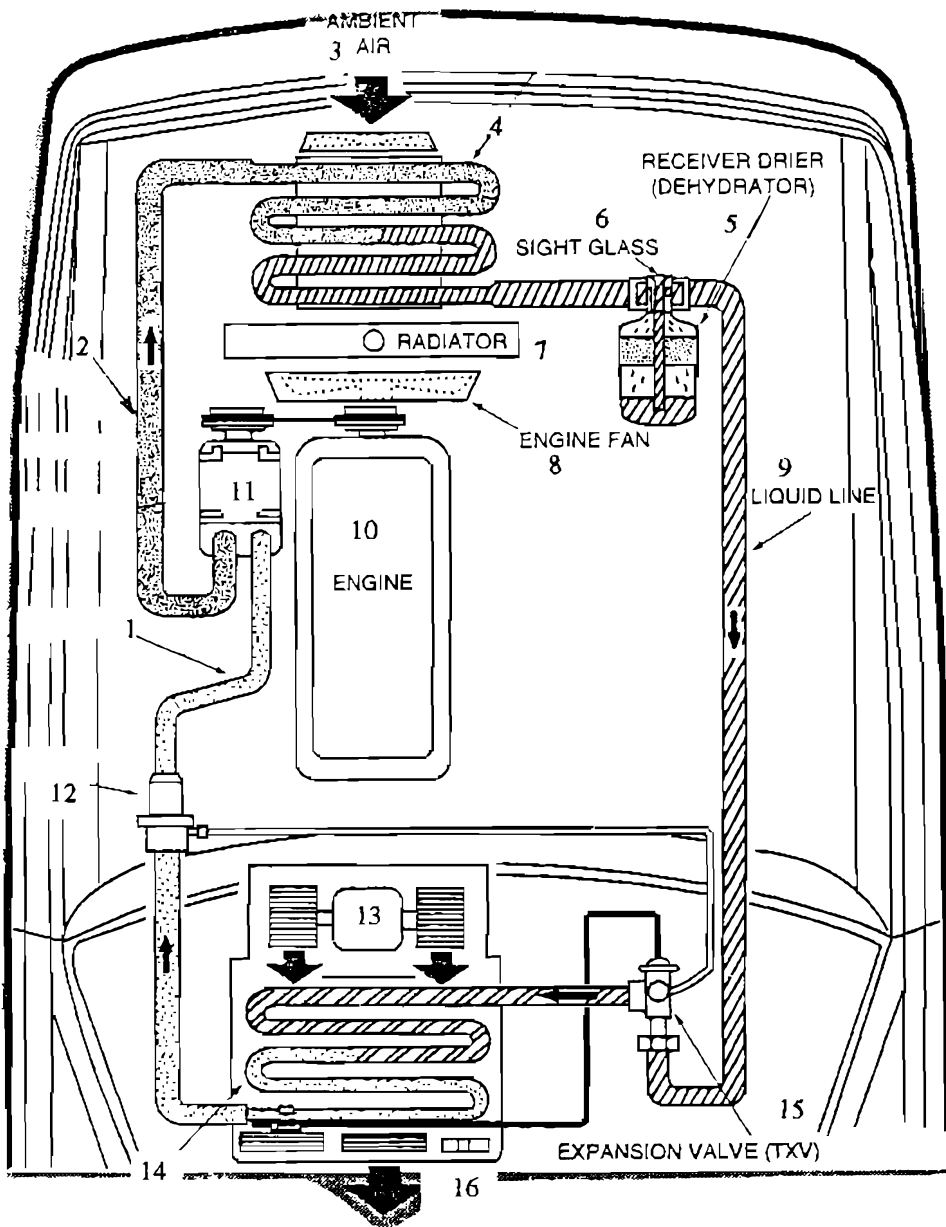
Hình 46. Các ống dẫn môi chất trên hệ thống điện lạnh ô tô trang bị van giãn nở: 1. Ống hút về môi chất thể hơi thấp áp. 2. Ống bơm đi môi chất thể hơi cao áp. 3. Không khí nóng ngoài xe. 4. Giàn nóng. 5. Bầu lọc / hút ẩm. 6. Mắt ga. 7. Kết nước làm mát động cơ. 8. Quạt kết nước. 9. Ống dẫn môi chất lỏng cao áp. 10. Động cơ. 11. Máy nén. 12. Van STV điều tiết hơi môi chất trở về máy nén. 13. Quạt lồng sóc. 14. Giàn lạnh. 15. Van giãn nở. 16. Không khí lạnh.
