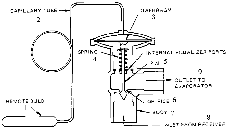
Hình 38. Kết cấu của van giãn nở trang bị bầu cảm biến nhiệt độ : 1. Bầu cảm biến nhiệt độ. 2. Ống mao dẫn. 3. Màng tác động. 4. Lò xo. 5. Chốt van. 6. Lỗ tiết lưu thay đổi. 7. Thân van. 8. Môi chất lạnh lỏng từ bầu lọc đi vào. 9. Cửa ra của môi chất lạnh lỏng phun vào bộ bốc hơi.
