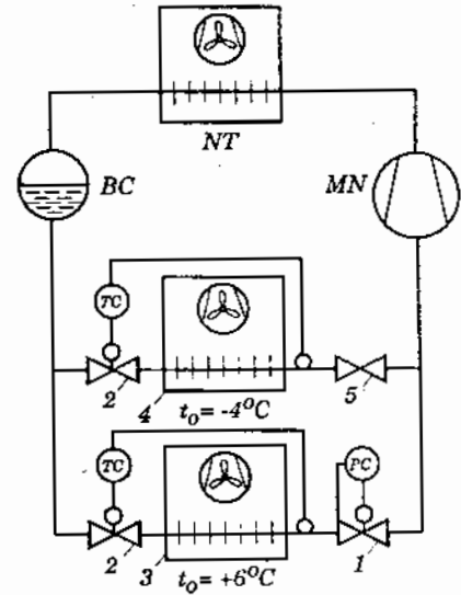
Hình 9.11. Ứng dụng đơn giản của van điều chỉnh áp suất bay hơi
