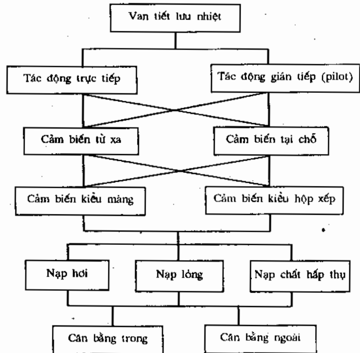
Hình 10.23. Phân loại van tiết lưu nhiệt.
