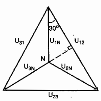
Hình 1.46. Các loại điện áp ngoài (điện áp dây).
