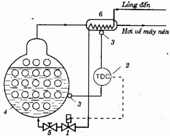
Hình 6.9. Cấp lỏng cho bình bay hơi freon, lấy tín hiệu nhiệt độ quá nhiệt tại bộ hồi nhiệt : 1 - van điện từ ; 2 - role hiệu nhiệt độ ; 3 - đầu cảm nhiệt ; 4 - bình bay hơi ; 5 - van tiết lưu tay ; 6 - hồi nhiệt.
