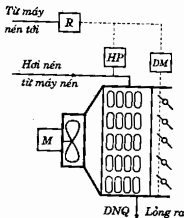
Hình 5.15. Sơ đồ điều chỉnh clapê gió để điều chỉnh nhiệt độ và áp suất ngưng tụ : HP - Role áp suất cao DM - Động cơ điều chỉnh clapê (Damper Motor) R - Contactor DNQ - Dàn ngưng quạt M - Động cơ quạt (Motor).
