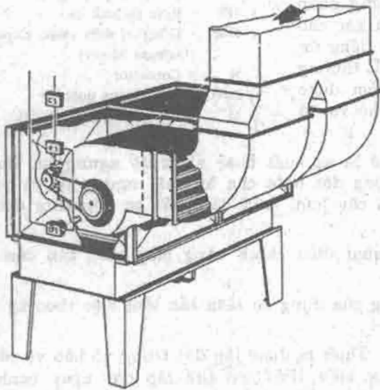
Hình 5.14. Hình ảnh bố trí rơle nhiệt độ điều khiển đóng ngắt quạt li tâm dàn ngưng để điều chỉnh nhiệt độ ngưng tụ.
