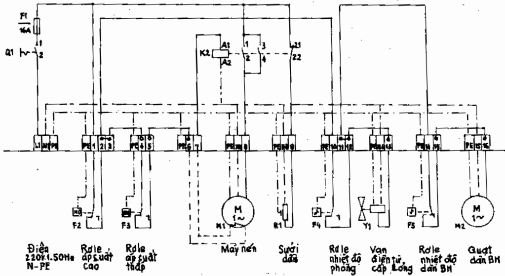
Hình 2.74. Sơ đồ mạch chính, mạch điều khiển và thanh kẹp của một hệ thống lạnh được sản xuất hàng loạt (Fischer - CHLB Đức)
