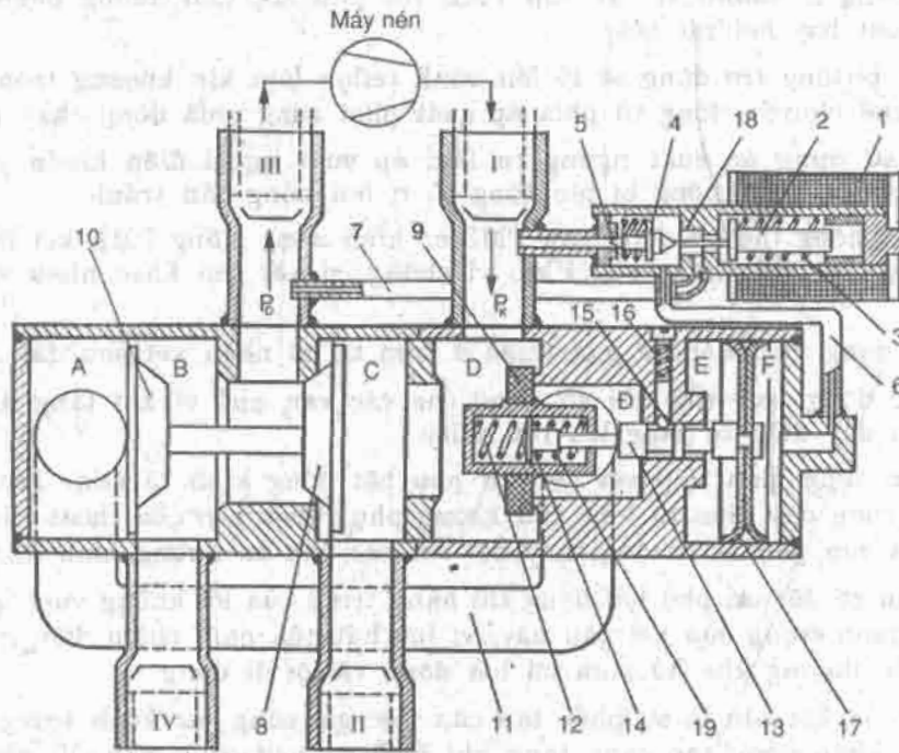
Hình 8.10. Van điện từ chuyển dòng 4 ngã APR :
