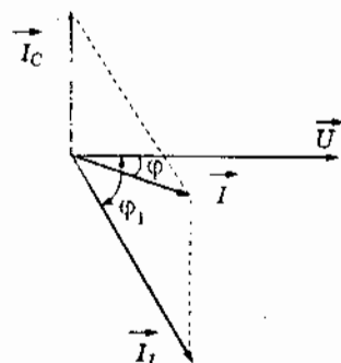
Hình 1.44. Dòng điện tổng hợp I từ I_c và I_1 .
