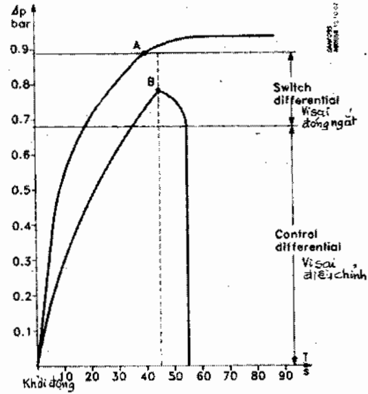
Hình 9.8. Đặc tính làm việc của role hiệu áp dầu khi máy nén khởi động.
