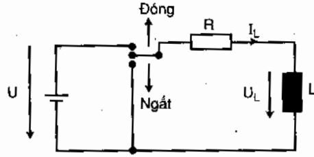
Hình 1.36. Sơ đồ thí nghiệm tính chất đóng ngắt cuộn dây.
