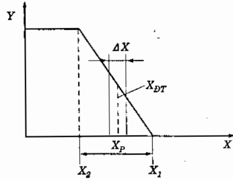
Hình 3.11. Đặc tính của điều chỉnh tỷ lệ :
