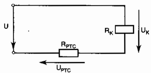
Hình 1.13. Mạch đơn giản.
