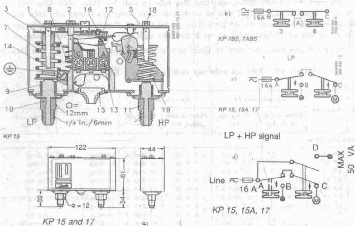
Hình 9.5. Cấu tạo của role áp suất kép kiểu KP15 của Danfoss:
