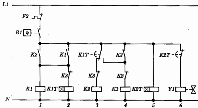
Hình 2.52. Mạch điện khởi động Y - Δ với van điện từ giảm tải máy nén Y1.
