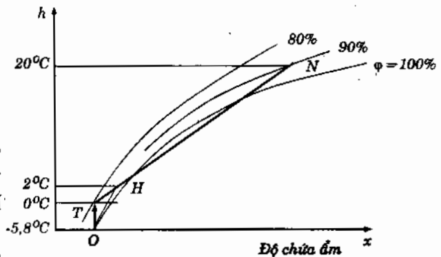
Hình 7.18. Hòa trộn không khí buồng lạnh và ngoài trời.
