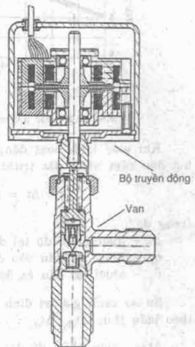
Hình 10.27. Van tiết lưu điện tử kiểu RTC của Engelhof.
