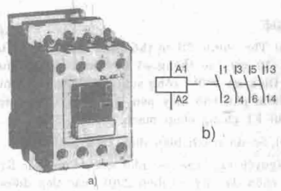
Hình 2.2. Contactor (hãng SCHIELE CHEB Đức) kiểu DLAK-10 ;
