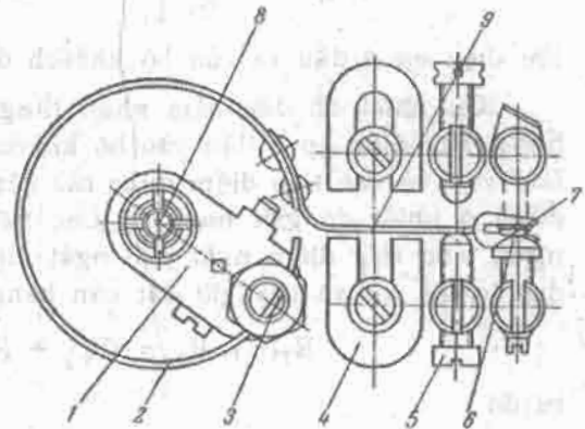
Hình 10.12. Nguyên tắc cấu tạo rơle nhiệt độ dẫn nở nhiệt bằng thanh lưỡng kim ký hiệu ĐTKB của Nga:
