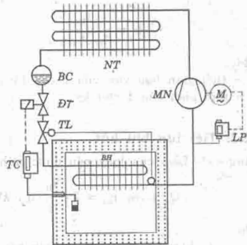
Hình 4.2. Điều chỉnh năng suất lạnh hai vị trí gián tiếp qua rơle áp suất thấp LP (Low Pressure Switch) : DT - Van điện từ ; BC - Bình chứa cao áp ; TL - Van tiết lưu nhiệt (các ký hiệu khác như hình 4.1).
