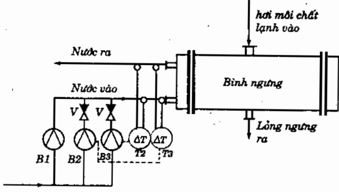
Hình 5.8. Sơ đồ điều chỉnh lưu lượng nước ngưng tụ bằng role hiệu nhiệt độ : B1, B2, B3 - Bơm 1, 2, 3 ; T2, T3 - Role hiệu nhiệt độ ; V - Van 1 chiều.
