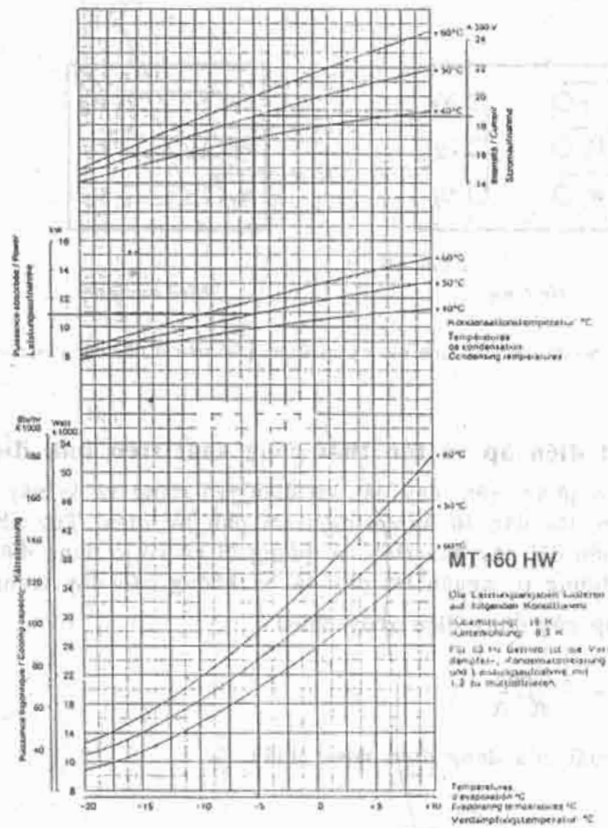
Hình 1.54. Catalog máy nén MT160HW của Maneurop.
