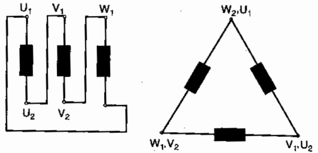
Hình 1.19. Mạng đầu hình tam giác \Delta .
