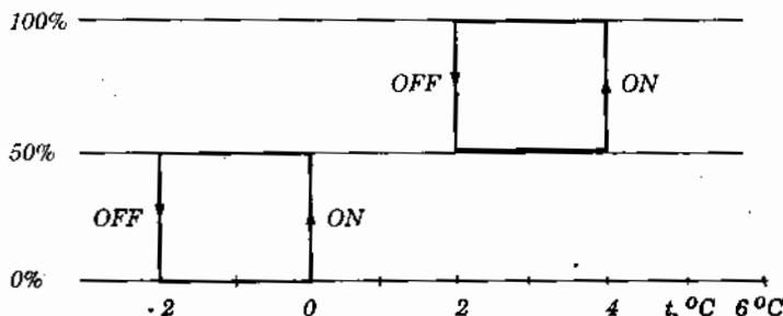
Hình 3.9. Đặc tính điều chỉnh 3 cấp, vị sai \Delta X = 2\text{K} .
