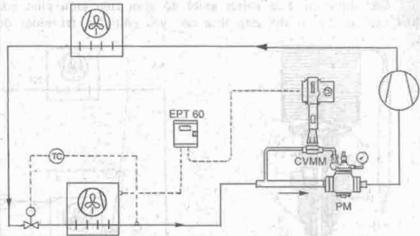
Hình 10.19. Sử dụng tổ hợp PM + CVMM + EPT 60 để điều chỉnh nhiệt độ buồng lạnh.
