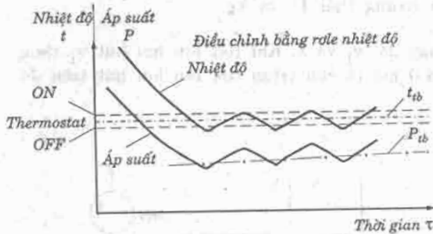
Hình 4.3. Đặc tính nhiệt độ buồng lạnh và áp suất bay hơi tương ứng hình 4.1.
