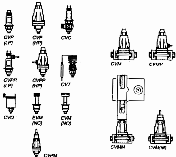
Hình 8.14. Các loại van pilot cho van chủ PM
