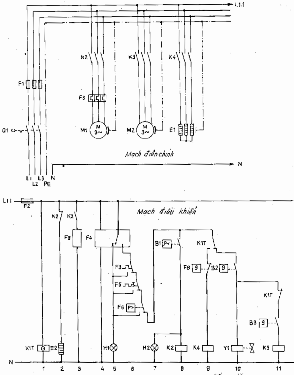
Hình 2.77. Mạch điều khiển hình 2.76 vẽ lại theo mạch khai triển :
