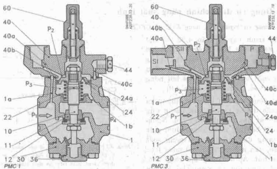
Hình 9.19. Van chủ PMC1 và PMC3 :
