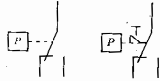
Hình 2.41. Ký hiệu mạch điện role áp suất :
