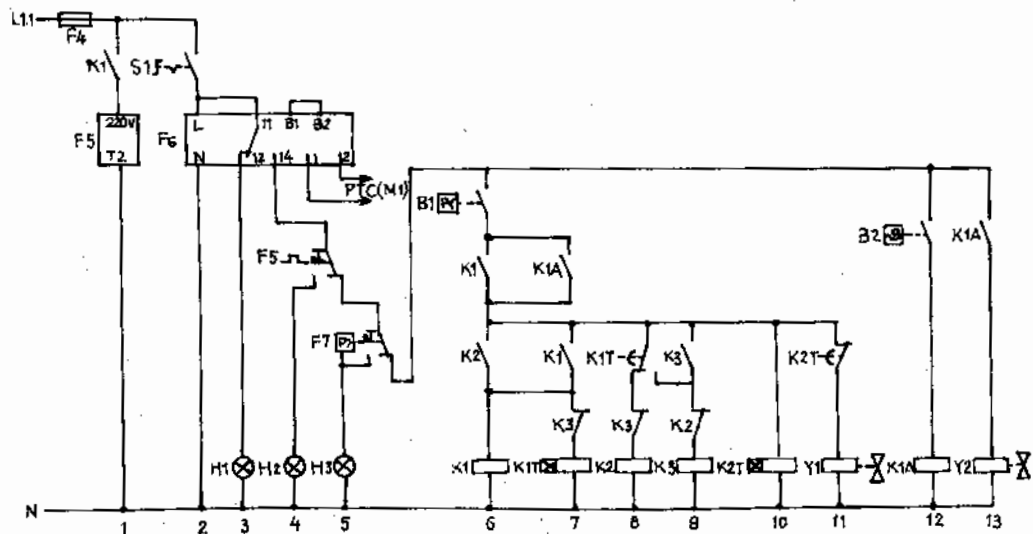
Hình 2.62. Mạch chính và mạch điều khiển thí dụ 2.13 :
