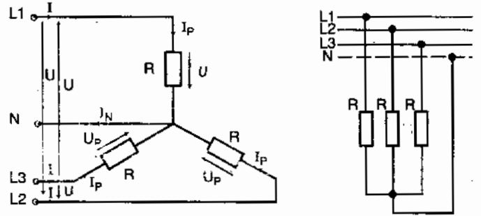
Hình 1.48. Điện trở thuần mắc hình sao :
