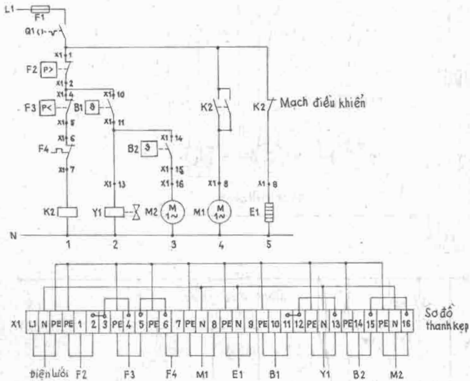
Hình 2.75. Sơ đồ mạch điều khiển và thanh kẹp.
