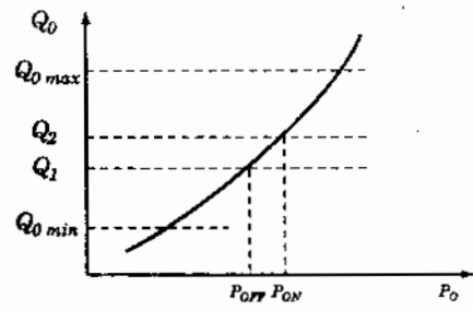
Hình 7.12. Đặc tính năng suất lạnh theo áp suất hút và điểm đóng ngắt của role áp suất điều khiển van điện tử P_{ON} , P_{OFF} .
