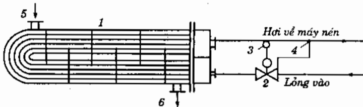
Hình 6.10. Cấp lỏng bình bay hơi lỏng sôi trong ống bằng van tiết lưu nhiệt cân bằng ngoài : 1 - bình bay hơi lỏng sôi trong ống ; 2 - van tiết lưu nhiệt cân bằng ngoài ; 3 - đầu cảm nhiệt ; 4 - đầu lấy tín hiệu áp suất ; 5, 6 - ống chất tải lạnh vào và ra.
