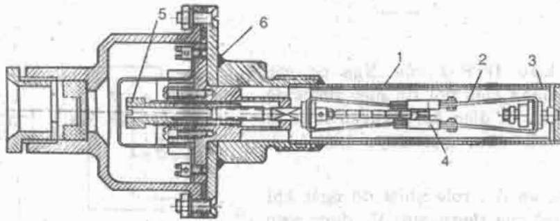
Hình 10.11. Cấu tạo của rơle nhiệt độ kiểu dẫn nở nhiệt hai phần tử TP200 (Nga);
