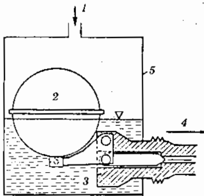
Hình 11.17. Một loại van phao cao áp : 1 - lồng tử dàn ngưng ; 2 - phao ; 3 - đế và kim van ; 4 - lồng đến dàn bay hơi ; 5 - vỏ phao.
