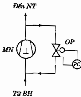
Hình 4.9. Bypass xả hơi nén về đường hút có bố trí van ổn áp OP :
