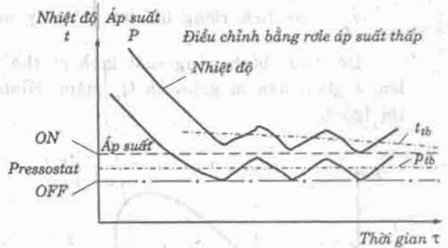
Hình 4.4. Đặc tính nhiệt độ buồng lạnh và áp suất bay hơi tương ứng hệ thống lạnh hình 4.2.
