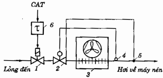
Hình 6.18. Sơ đồ bảo vệ dàn bay hơi không bị tràn lỏng :
