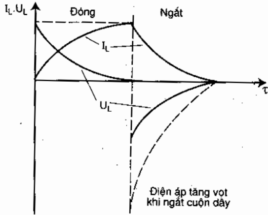
Hình 1.37. Tính chất đóng và ngắt cuộn dây.
