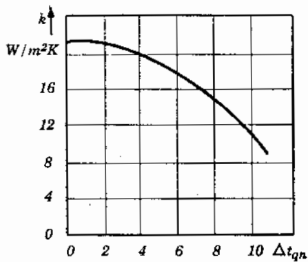
Hình 6.1. Sự phụ thuộc của hệ số truyền nhiệt k , W/m 2 K vào độ quá nhiệt hơi hút : \Delta t_{qn} = t_h - t_o , K ; t_h - nhiệt độ hơi hút ; t_o - nhiệt độ bay hơi,
