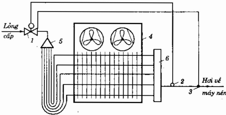
Hình 6.12. Cấp lỏng dàn bay hơi freôn lớn : 1 - van tiết lưu nhiệt cân bằng ngoài ; 2 - đầu cảm nhiệt ; 3 - ống lấy tín hiệu áp suất hút ; 4 - dàn lạnh quạt ; 5 - đầu chia lỏng ; 6 - ống góp hơi.
