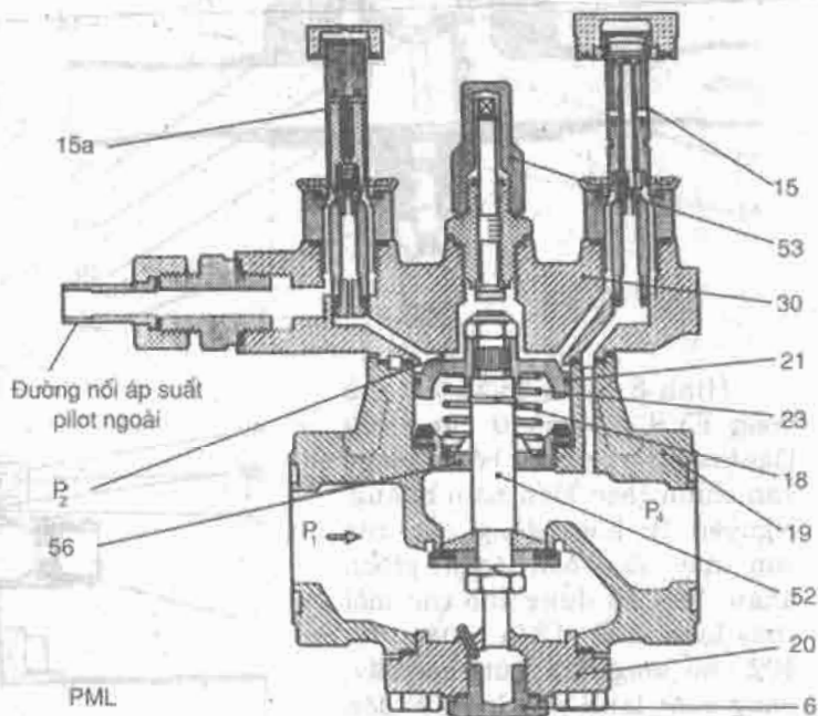
Hình 8.7. Van điện tử trợ động PML của Danfoss;
