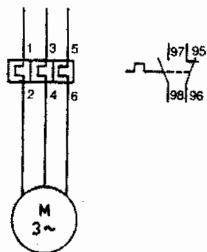
Hình 2.29. Ký hiệu role nhiệt trong mạch điện.
