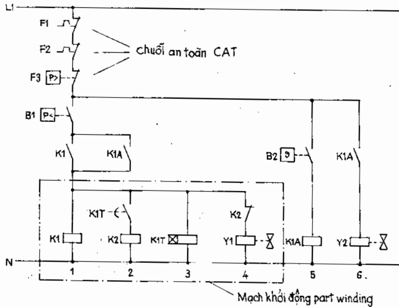
Hình 2.61. Máy nén với mạch khởi động part winding (một phần cuộn dây) và pump out.
