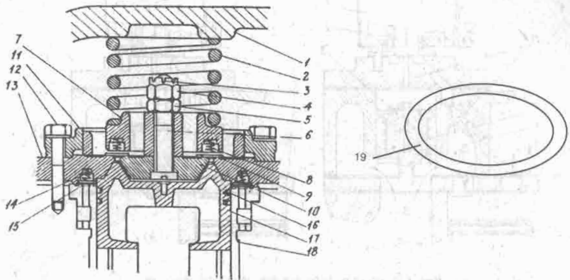
Hình 4.18. Dầu xi-lanh với cụm van hút và dấy kiểu vòng (MYCOM) :
