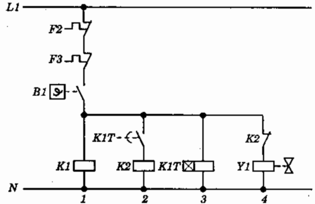
Hình 2.54. Mạch điều khiển khởi động part winding (một phần cuộn dây).
