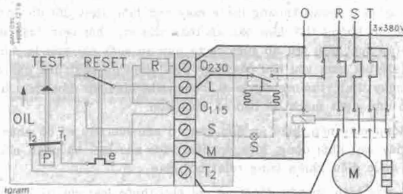
Hình 9.7. Sơ đồ mạch điện của rơle hiệu áp dầu lắp vào động cơ máy nén và điện trở sưởi cacte.
