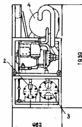
Hình 7.7b. Hình chiếu đứng và chiếu cạnh của Liquid chiller 30HK-100 :
