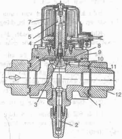
Hình 8.3. Van điện từ tác động gián tiếp có đế van phụ di động :
