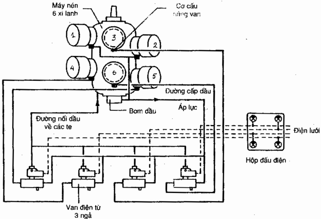
Hình 4.20. Sơ đồ hệ thống thủy lực điều khiển van điện tử để nâng van hút giảm tải và điều chỉnh năng suất lạnh của hãng Grasso (Hà Lan).
