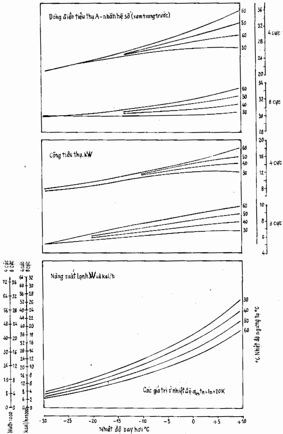
Hình 4.26. Tốc độ vòng quay và năng suất lạnh Q_0 của một máy nén BOCK ở 2 chế độ tốc độ khác nhau.
