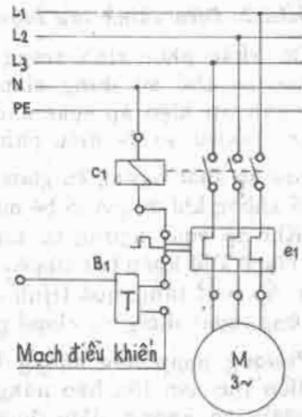
Hình 5.13. Sơ đồ mạch điều khiển quạt dàn ngưng có rơle nhiệt độ để điều chỉnh nhiệt độ và áp suất ngưng tụ : C1 - công tắc tơ động cơ ; e1 - rơle nhiệt ; B1 - rơle nhiệt độ.
