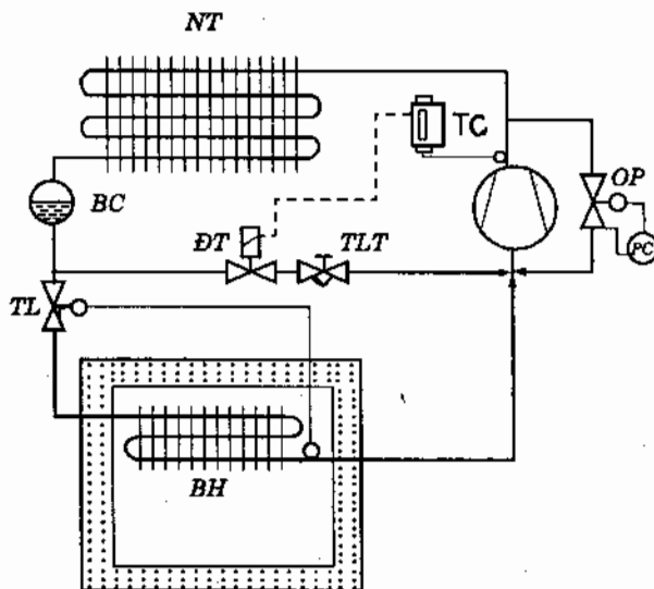
Hình 4.11. Xả hơi nén về đường hút, phun lỏng qua rơle nhiệt độ TC và van điện tử DT với van tiết lưu tay TLT.
