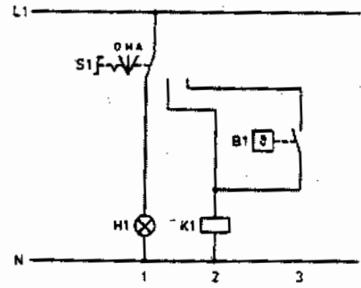
Hình 2.27. Mạch thiết kế cho thí dụ 2.7 với núm vặn 3 nấc : O = OFF H = Hand A = Auto S1 - Núm vặn 3 nấc H1 - Đèn hiệu "ngắt - OFF" B1 - Role nhiệt độ phòng K1 - Contactor máy nén.
