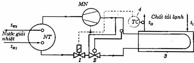
Hình 7.4. Máy lạnh freon, môi chất sôi trong ống, máy nén làm việc theo kiểu ON-OFF:
