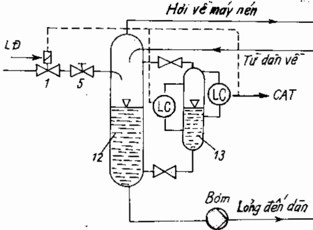
Hình 6.20. Sơ đồ bảo vệ bình chứa tuần hoàn amoniác; LD : bảo vệ liên động cùng máy nén ; CAT - chuỗi an toàn ; 12 - bình chứa tuần hoàn ; 13 - bình đo.
