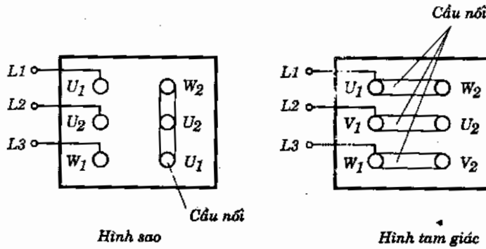
Hình 1.53. Sơ đồ đầu dây hình sao và hình tam giác trên ổ đầu dây của động cơ.
