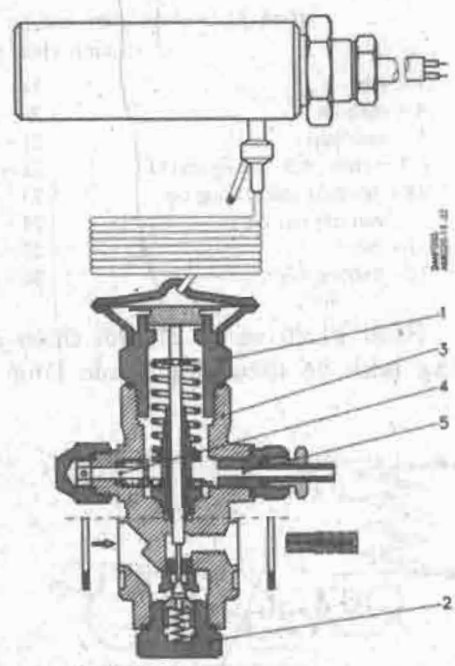
Hình 11.24. Van tĩnh nhiệt điều chỉnh mức lỏng TEVA 20 và TEVA 85 của Danfoss : 1 - phần tử tĩnh nhiệt (màng đàn hồi) ; 2 - cụm lỗ van ; 3 - thân van ; 4 - vít điều chỉnh (đặt) ; 5 - ống nối đường cân bằng áp suất ngoài.
