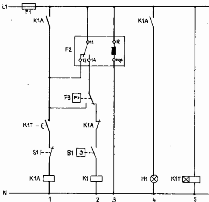
Hình 2.47. Mạch điều khiển an toàn cho reset và thermistor.
