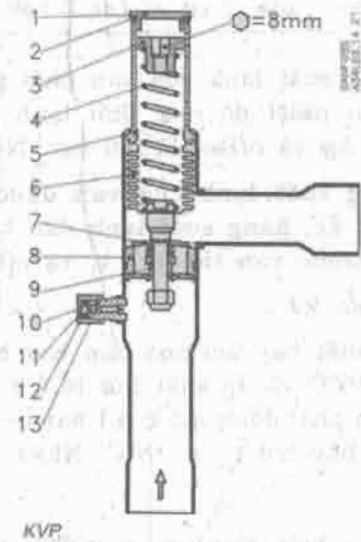
Hình 9.10. Kết cấu của van điều chỉnh áp suất bay hơi kiểu KVP của Danfoss :
