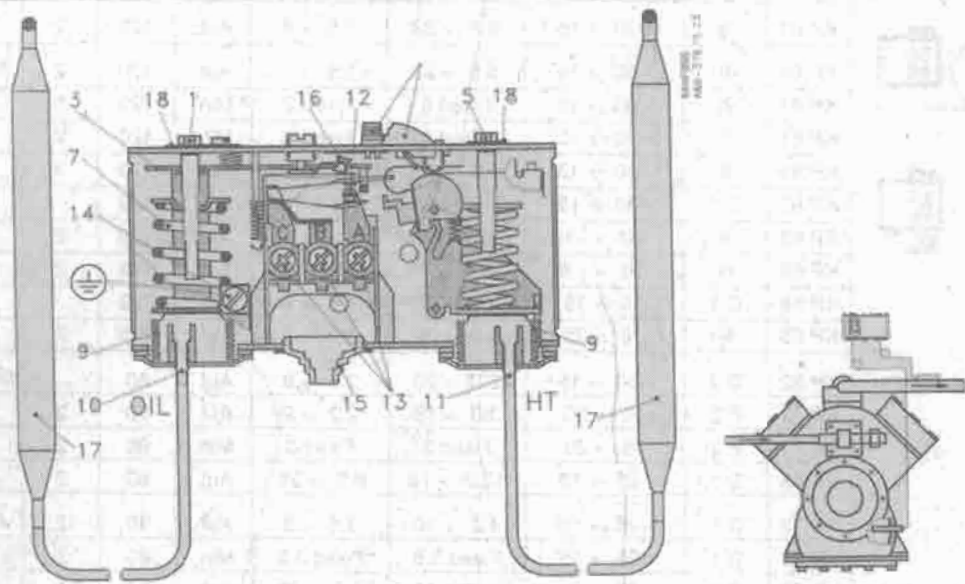
Hình 10.5. Role nhiệt độ đúp và ứng dụng bảo vệ nhiệt độ dầu máy không quá cao và nhiệt độ dầu không quá cao và không quá thấp :
