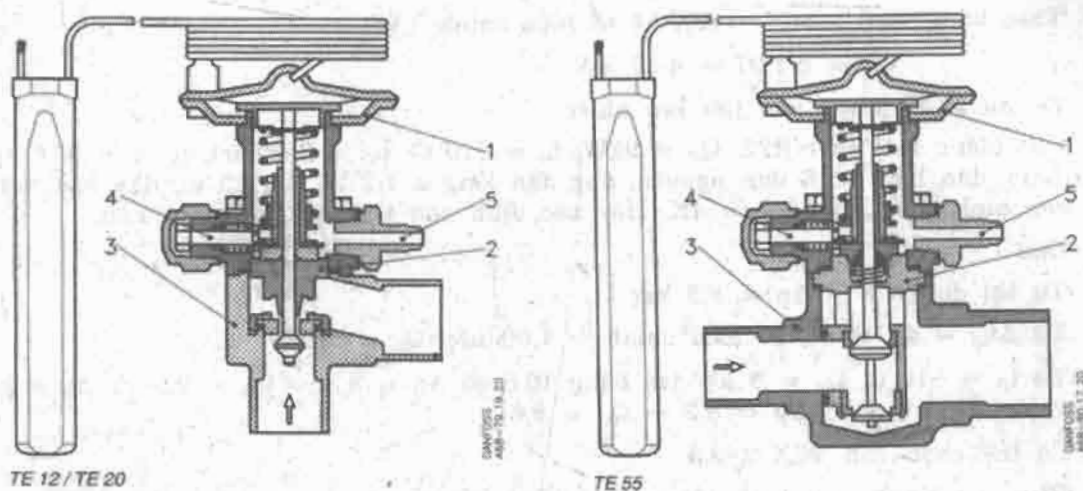
Hình 10.25. Cấu tạo van tiết lưu nhiệt kiểu TE 12/20 và TE 55 của Danfoss :
