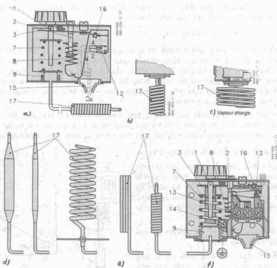
Hình 10.4. Cấu tạo rơle nhiệt độ hiệu KP của Danfoss :
