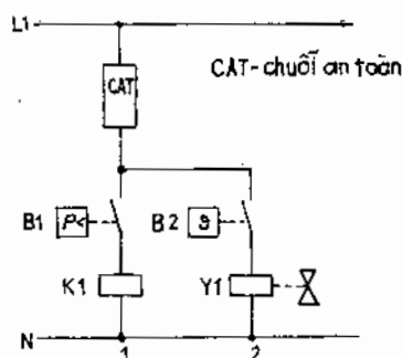
Hình 2.58. Mạch điều khiển pump down : B1 - role áp suất thấp B2 - Role nhiệt độ phòng K1 - Tiếp điểm máy nén Y1 - Van điện từ đường cấp lỏng.
