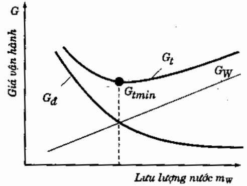
Hình 5.4. Cách tìm giá vận hành min từ giá điện và giá nước vận hành.
