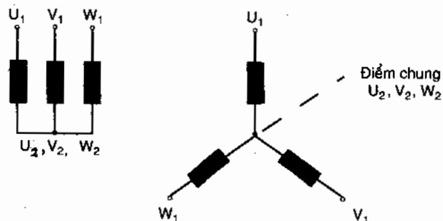
Hình 1.18. Mạch đấu hình sao.
