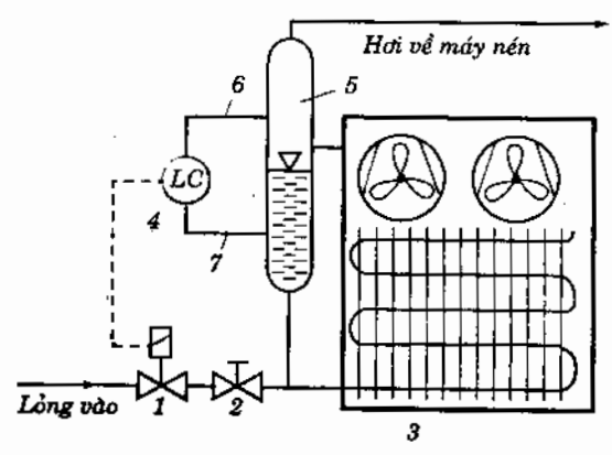
Hình 6.13. Cấp lỏng cho dàn bay hơi amoniác ; 1 - van điện từ ; 2 - van tiết lưu tay ; 3 - dàn bay hơi ; 4 - role mức lỏng (Level Controller) ; 5 - bình tách lỏng ; 7 - đường cân bằng lỏng.
