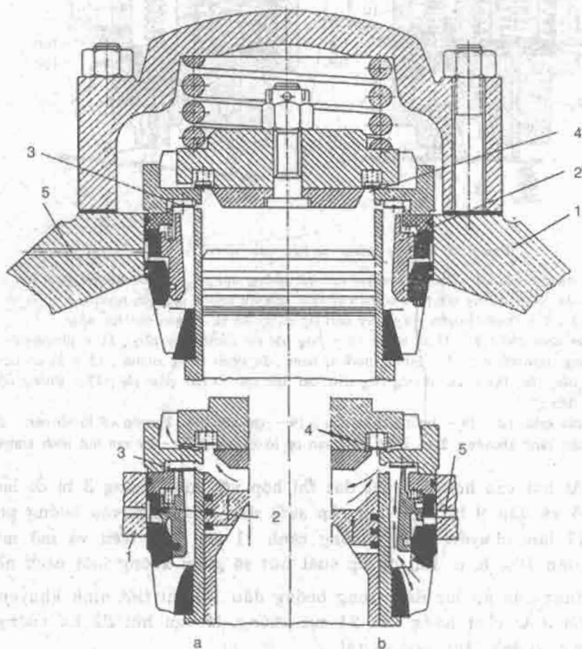
Hình 4.24. Cơ cấu nâng van của Brissoneau - Lotz : 1 - vòng dẫn hướng ; 2 - pittông phụ ; 3 - van hút ; 4 - van nén ; 5 - hơi nén vào.
