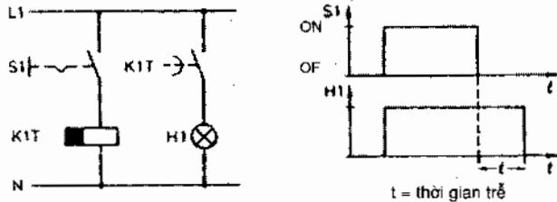
Hình 2.7. Role thời gian trễ nhà
