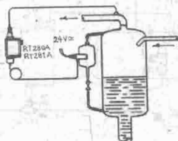
Hình 11.8. role mức lỏng RT 280/281A trong sơ đồ bảo vệ mức lỏng và báo động : Role ngắt máy nén và đóng mạch báo động.
