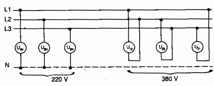
Hình 1.47. Biểu diễn phụ tải điện ba pha 220V và 380V 4 dây dẫn.
