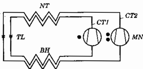
Hình 7.7. Nguyên tắc cấu tạo của Liquid chiller 30HK100-120 (Carrier) : CT1-CT2 - chu trình lạnh 1 và 2 ; MN - máy nén ; NT - bình ngưng tụ ; TL - van tiết lưu nhiệt ; BH - bình bay hơi.
