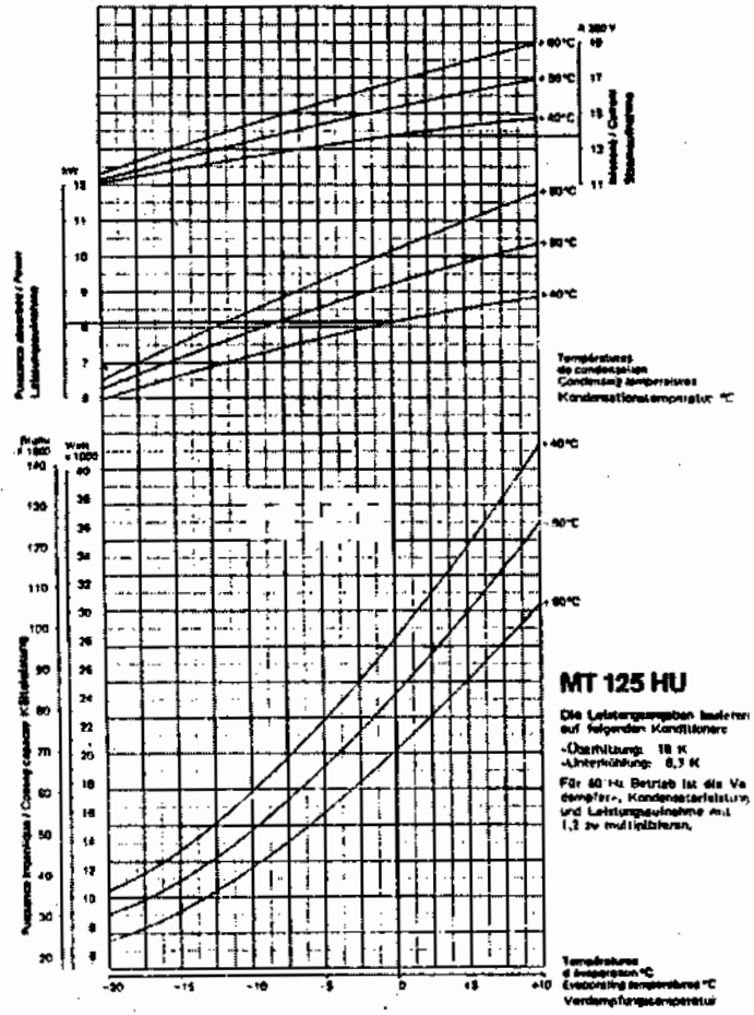
Hình 1.52. Đặc tính máy nén MT125HU hãng Maneurop (catalog của nhà chế tạo).
