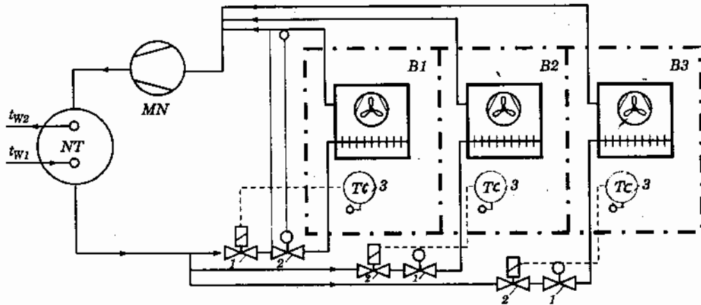
Hình 7.15. Máy lạnh với nhiều buồng lạnh xấp xỉ nhiệt độ 1 - van tiết lưu nhiệt cân bằng ngoài ; 2 - van điện từ ; 3 - role nhiệt độ.
