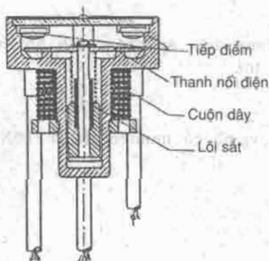
Hình 1.57. Một kiểu Role khởi động kiểu dòng điện (Danfoss) dùng cho các loại động cơ nhỏ (dưới 1 mã lực).
