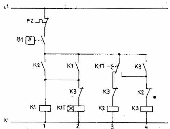
Hình 2.51. Mạch điện điều khiển của mạch khởi động \lambda - \Delta .
