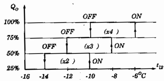
Hình 7.6. Thí dụ điều chỉnh năng suất lạnh với máy nén có 4 cụm xilanh : X1 ; X2 ; X3 ; X4, Q_o phụ thuộc vào nhiệt độ chất tải lạnh t_{12} .
