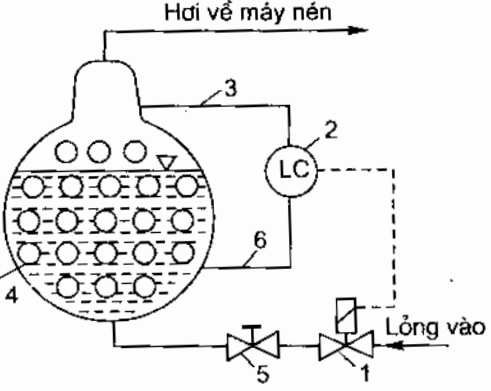
Hình 6.8. Cấp lỏng theo mức bằng điều chỉnh 2 vị trí :
