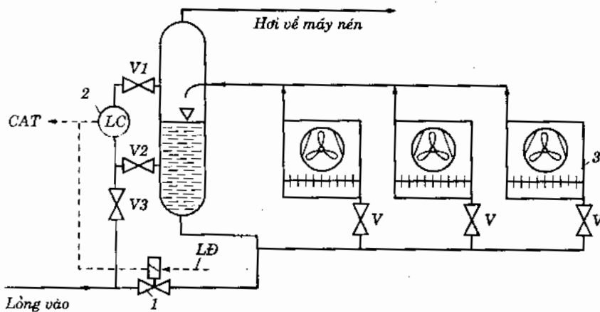
Hình 6.19. Sơ đồ bảo vệ tràn lỏng cho hệ thống dàn bay hơi amoniac :
