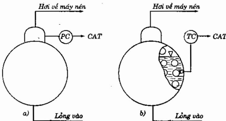
Hình 6.21. Sơ đồ bảo vệ bình bay hơi kiểu ngáp amoniác : (môi chất sôi trong không gian giữa các ống) khỏi bị đóng băng bằng chất tải lạnh trong ống : a) bằng rơle áp suất PC (Pressure Controller) ; b) bằng rơle nhiệt độ (Temperature controller).
