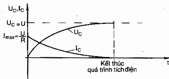
Hình 1.27. Biến thiên điện thế U_C và cường độ I_C của tụ theo thời gian trong quá trình tích điện.
