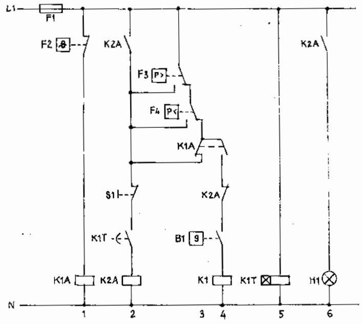
Hình 2.48. Mạch điều khiển thí dụ 2.10.
