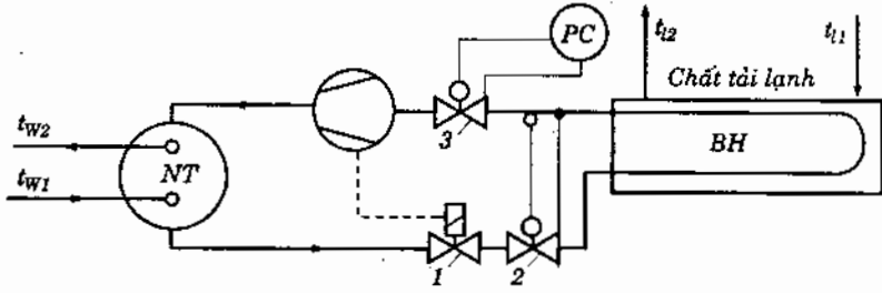
Hình 7.13. Sơ đồ điều chỉnh năng suất lạnh theo áp suất sôi : 1 - van điện tử ; 2 - van tiết lưu nhiệt ; 3 - van điều chỉnh áp suất bay hơi tự động.
