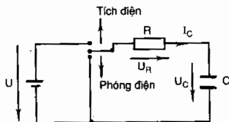
Hình 1.26. Mạch thí nghiệm tính chất tích và phóng điện của tụ.
