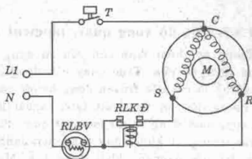
Hình 1.56. Sơ đồ điện động cơ một pha đơn giản chỉ có role khởi động RLKD và role bảo vệ :
