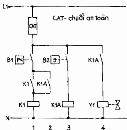
Hình 2.59. Mạch điều khiển pump out K1A - tiếp điểm phụ. (các kí hiệu khác như h.2.57)
