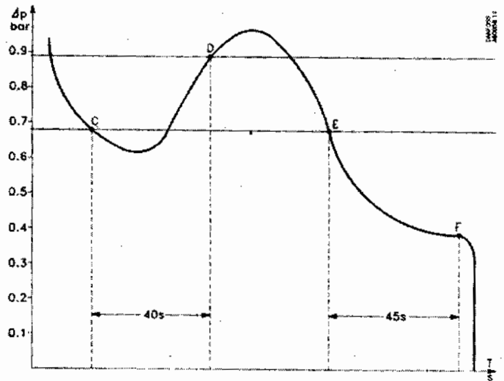
Hình 9.9. Đặc tính làm việc của role hiệu áp dầu khi máy nén đang vận hành.
