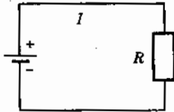
Hình 1.7. Mạch điện.
