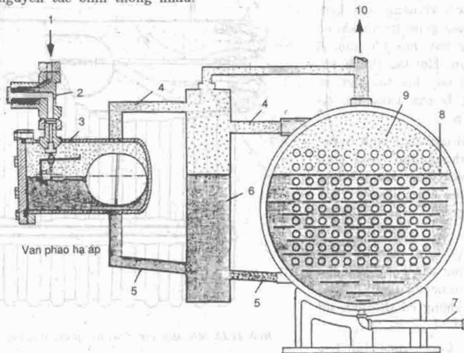
Hình 11.10. Nguyên tắc cấu tạo và làm việc của van phao hạ áp điều chỉnh liên tục mức lỏng cho bình bay hơi kiểu ngập :
