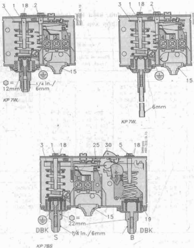
Hình 9.4. Role áp suất cao kiểu KP7W của Danfoss :
