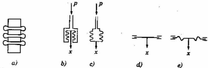
Hình 9.1. Các phần tử cảm biến đàn hồi:
