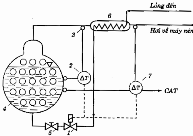
Hình 6.17. Sơ đồ bảo vệ bình bay hơi ống vỏ kiểu ngập freon không bị tràn lỏng :
