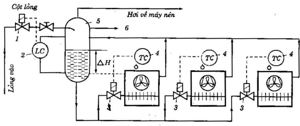
Hình 6.14. Sơ đồ cấp lỏng cho nhiều dàn bay hơi nhờ cột lỏng : 1 - van điện từ cấp lỏng ; 2 - role mức lỏng kiểu phao ; 3 - van điện từ điều chỉnh nhiệt độ buồng lạnh ; 4 - role nhiệt độ điều chỉnh nhiệt độ buồng lạnh ; 5 - bình tách lỏng ; 6 - ống chảy tràn về bình chứa.
