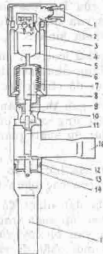
Hình 10.21. Cấu tạo của van điện tử KVQ của Danfoss
