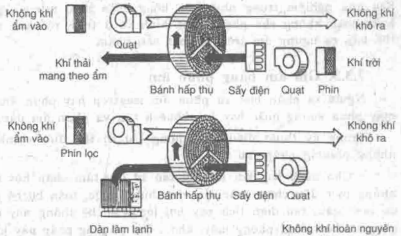
Hình 7.20. Máy hút ẩm bằng hấp thụ của MUNTERS (Hai phương pháp hoàn nguyên).
