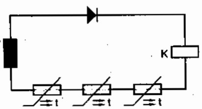
Hình 1.12. Mạch bảo vệ động cơ thermistor : K – Role.
