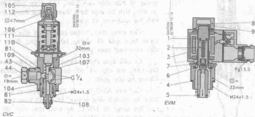
Hình 9.20. Van pilot CVC:
