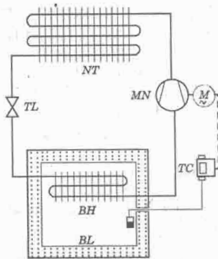
Hình 4.1. Máy nén lạnh dùng rơle nhiệt độ trực tiếp đóng ngắt máy nén : MN - Máy nén ; M - Động cơ (Motor) máy nén ; NT - Dàn ngưng tụ ; TL - Tiết lưu (ống mao dẫn) ; BH - Dàn bay hơi ; BL - Buồng lạnh cách nhiệt ; TC - Rơle nhiệt độ (Thermostat). (TC = Temperature Control).
