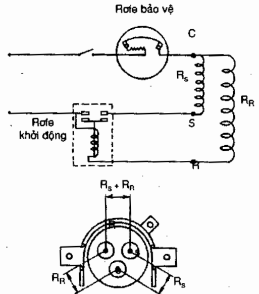
Hình 1.16. Sơ đồ cuộn dây của máy nén kín (block) hãng Danfoss :
