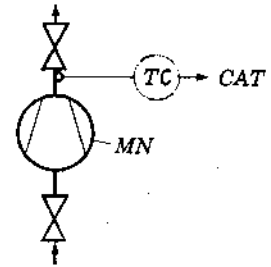
Hình 4.32. Khống chế nhiệt độ dầu dầy bằng role nhiệt độ : TC- role nhiệt độ (thermostat) ; CAT - chuỗi an toàn.
