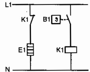
Hình 2.19. Sơ đồ mạch điện bộ sưởi dầu.
