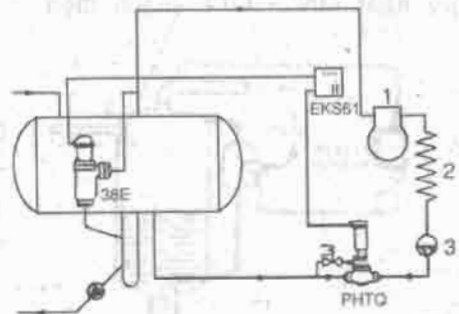
Hình 11.6. Kết hợp hộp phao 38E với EKS 61 và PHTQ để điều chỉnh mức lỏng phía hạ áp :
