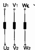
Hình 1.17. Ký hiệu 3 cuộn dây của động cơ ba pha.
