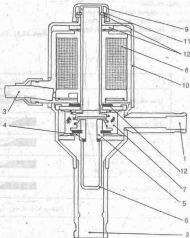
Hình 10.30. Cấu tạo van tiết lưu điện tử kiểu AKV.
