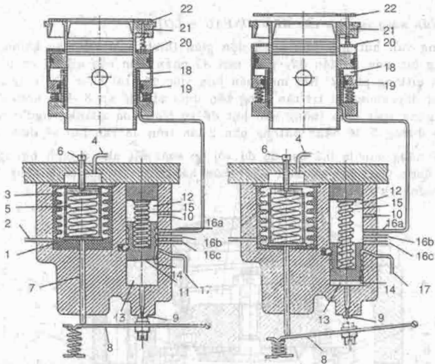
Hình 4.23. Cơ cấu nâng van hút của TRANE :
