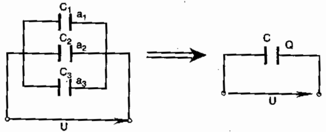
Hình 1.23. Mạch tụ điện song song.
