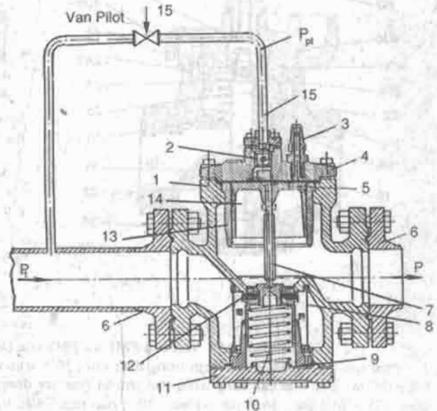
Hình 8.12. Van thừa hành pilot, van lái với van chủ: 1 - thân van ; 2 - bộ lọc ; 3 - vít mở van bằng tay ; 4 - nắp trên ; 5 - lỗ cân bằng ; 6 - bích nối ; 7 - thanh dây ; 8 - ống lưới lọc ; 9 - ống dẫn hướng ; 10 - lò xo ; 11 - nắp dưới ; 12 - tấm van ; 13 - xilanh ; 14 - pittông ; 15 - van pilot.
