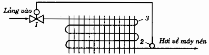
Hình 6.11. Cấp lỏng cho dàn bay hơi freôn bằng van tiết lưu nhiệt cân bằng trong : 1 - van tiết lưu nhiệt cân bằng trong ; 2 - đầu cảm nhiệt ; 3 - dàn bay hơi.
