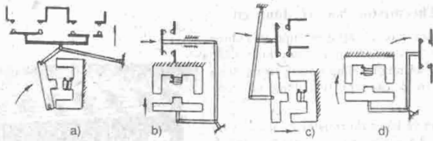
Hình 2.33. Nguyên tắc cấu tạo Contactor điện từ điện xoay chiều :
