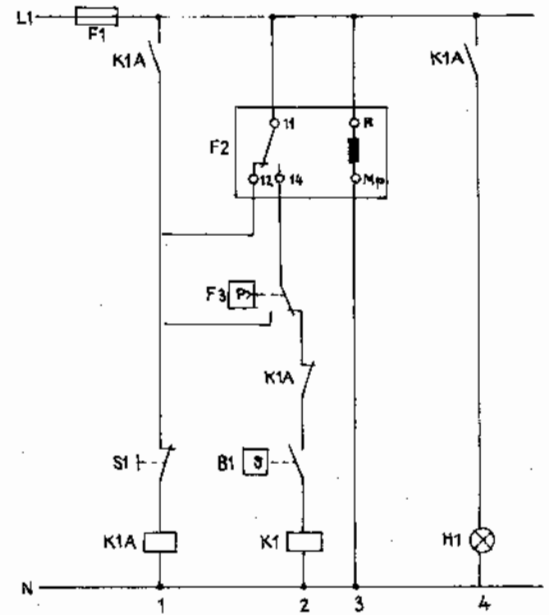
Hình 2.46. Đèn báo chung với reset và một khí cụ điện làm việc theo nguyên tắc dòng điện tĩnh.
