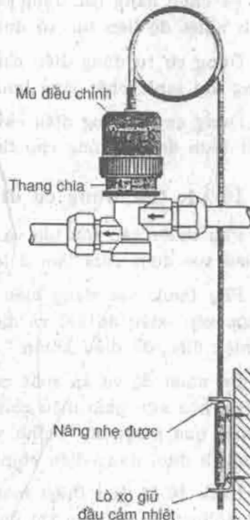
Hình 10.15. Van điều chỉnh nhiệt độ liên tục.
