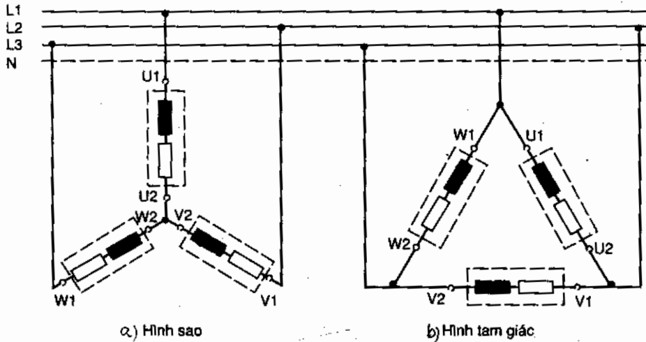
Hình 1.51. Động cơ máy nén mắc vào lưới điện 3 pha. a) Hình sao ; b) Hình tam giác
