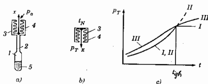
Hình 10.1. Sơ đồ nguyên lý hệ thống biến đổi nhiệt áp từ xa (a) và tại chỗ (b) cũng như đặc tính nhiệt độ - áp suất hơi I (c) t_N - nhiệt độ bên ngoài ; p_i - áp suất bên trong đầu cảm nhiệt ; p_a - áp suất môi trường bên ngoài ; x - độ dịch chuyển cơ học ; 1 - đầu cảm nhiệt ; 2 - ống mao dẫn tín hiệu áp suất ; 3 - hộp xếp ; 4 - vỏ ngoài hộp xếp ; 5 - chất lỏng.
