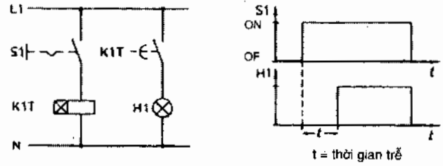
Hình 2.6. Role thời gian trễ hút
