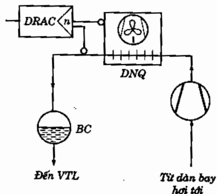
Hình 5.16. Sơ đồ điều chỉnh vô cấp quạt dàn ngưng tụ bằng máy biến tần của hãng Danfoss : DRAC - Máy biến tần DRAC của Danfoss DNQ - Dàn ngưng quạt.
