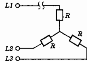
Hình 1.50. Mất pha L1 không nối N.
