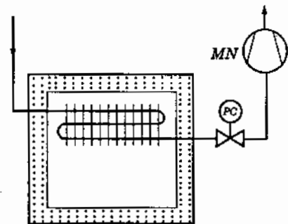
Hình 4.7. Sơ đồ thiết bị chu trình tiết lưu hơi hút PC - Van ổn áp và điều chỉnh áp suất hút theo năng suất lạnh yêu cầu.
