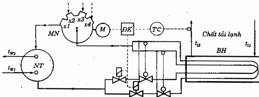
Hình 7.5. Máy lạnh freon với bình bay hơi môi chất sôi trong ống, máy nén ngắt từng cụm xilanh: TC- role nhiệt độ; ĐK - mạch điều khiển.
