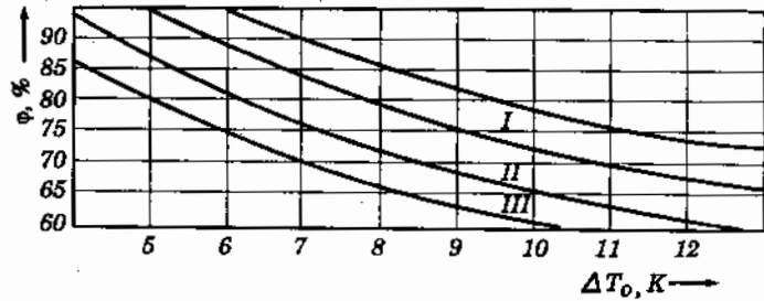
Hình 7.17. Xác định độ ẩm và hiệu nhiệt độ \Delta t_o cho các loại buồng lạnh khác nhau theo hãng Roller : I - Đối với sản phẩm bảo quản đòi hỏi độ ẩm thấp II- Đối với sản phẩm bảo quản đòi hỏi độ ẩm trung bình III- Đối với sản phẩm bảo quản đòi hỏi độ ẩm cao (Nên chọn định hướng ở giữa vùng II).
