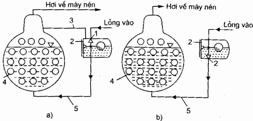
Hình 6.7. Cấp lỏng cho bình bay hơi bằng van phao : a) Hạ áp ; b) Cao áp. 1 - van tác động nhờ phao ; 2 - buồng phao ; 3 - đường cân bằng hơi ; 4 - bình bay hơi ; 5 - đường cân bằng lỏng.
