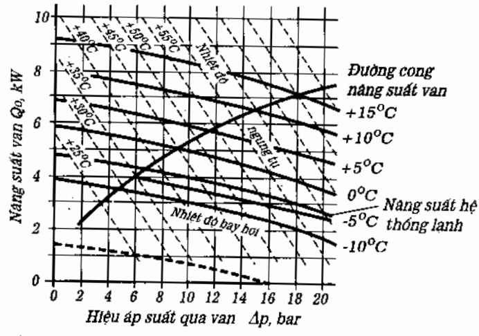
Hình 5.2. Đường cong năng suất van với các đường cong nhiệt độ ngưng tụ và nhiệt độ bay hơi.
