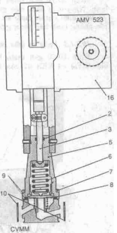
Hình 10.18. Van pilot CVMM :
