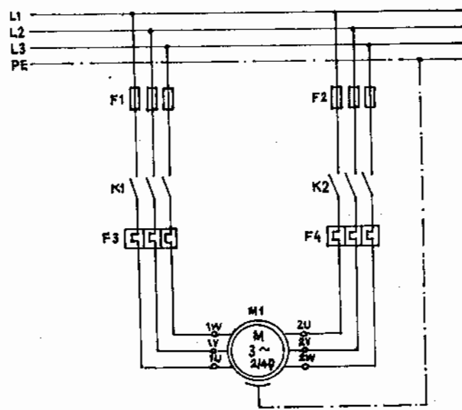
Hình 2.69. Mạch chính của một động cơ 2 tốc độ với các cuộn dây riêng biệt.
