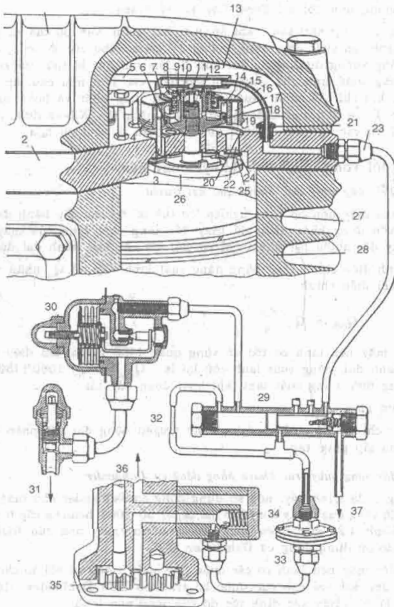
Hình 4.25. Cơ cấu rỗng van của Stal :
