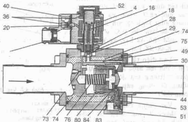
Hình 8.6. Van điện tử tự động EVR 32 và 40 của Danfoss kiểu thường đóng NC (chú thích xem hình 8.5).
