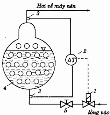
Hình 6.6. Sơ đồ cấp lỏng theo độ quá nhiệt cho bình bay hơi kết hợp với dụng cụ điều chỉnh 2 vị trí :
