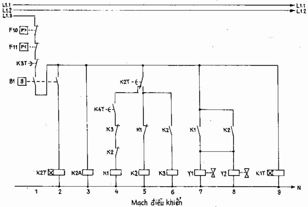
Hình 2.73. Mạch chính và mạch điều khiển của máy nén trực vít với động cơ Dahlander 2 tốc độ :
