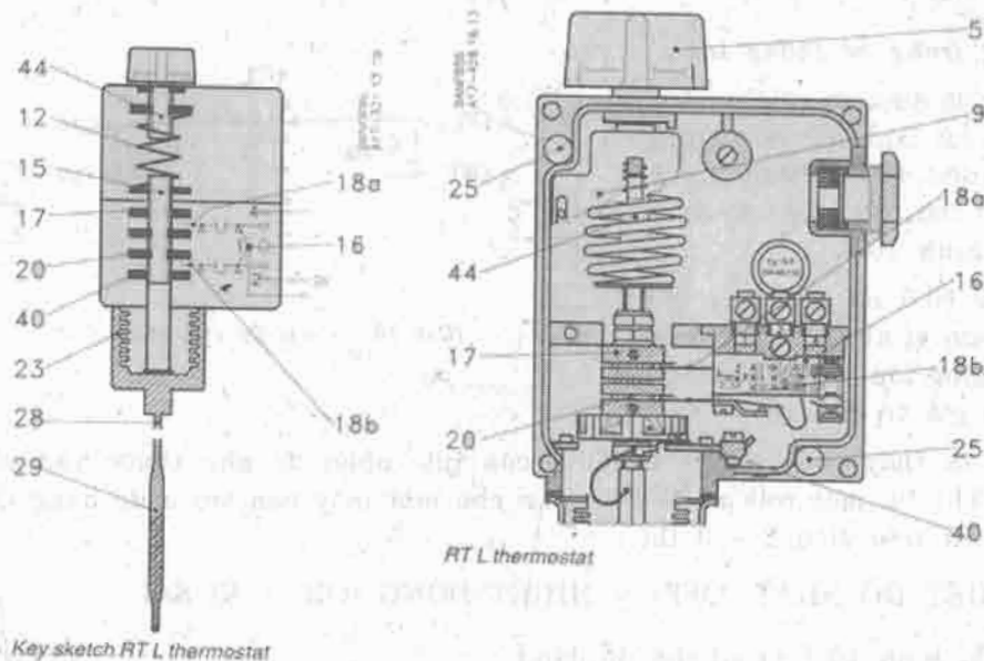
Hình 10.8. Role nhiệt độ RTL của Danfoss :
