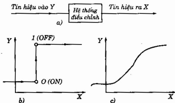
Hình 3.10. So sánh giá trị điều chỉnh 2 vị trí và liên tục :
