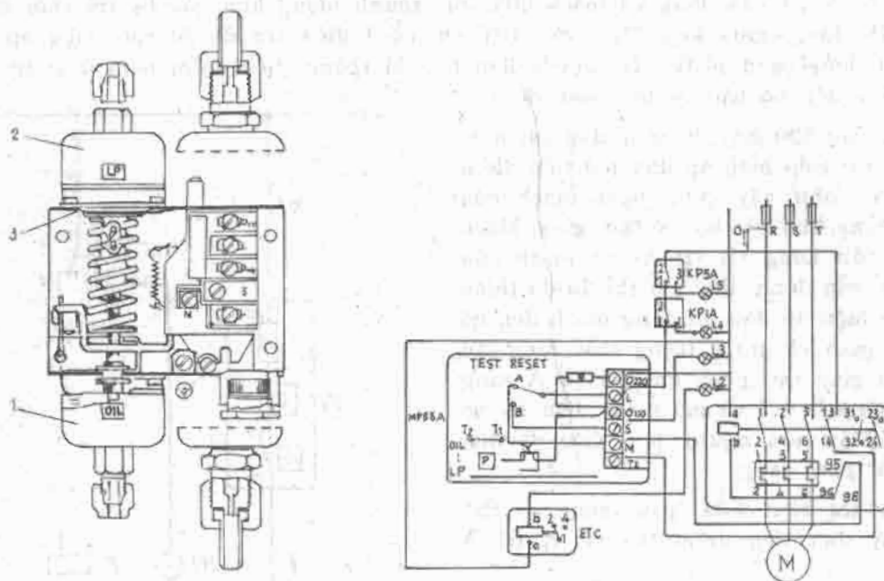
Hình 2.38. Rơle hiệu áp dầu và sơ đồ nguyên lý mạch điện (Danfoss).
