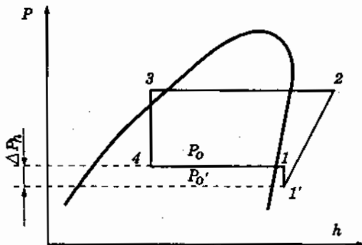
Hình 4.6. Chu trình tiết lưu hơi hút biểu diễn trên đồ thị lgp-h : 1-1' : quá trình tiết lưu hơi hút từ p_o xuống p_o' .
