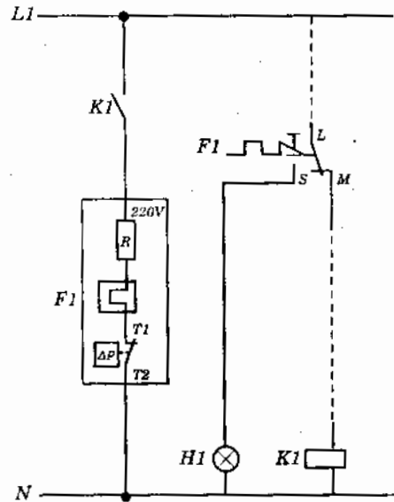
Hình 2.40. Biểu diễn mạch điện của role hiệu áp dầu trên sơ đồ điện.
