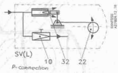
Hình 11.23. Sơ đồ mắc song song đường cấp lỏng qua van phao và qua van tiết lưu tay (nút 11 và ống C như hình 11.13 và 11.9 ; tháo vít 25).
