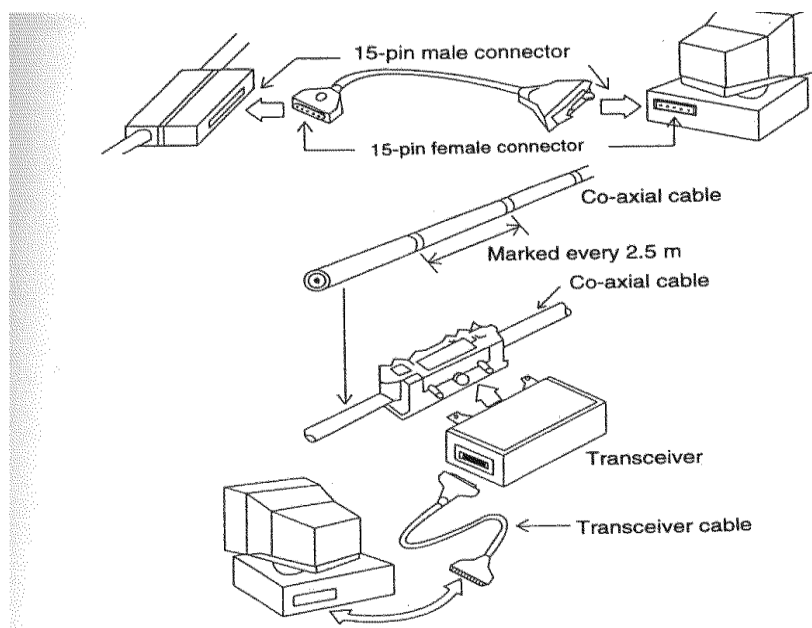
Hình 4.3: Kết nối bằng Traceiver
